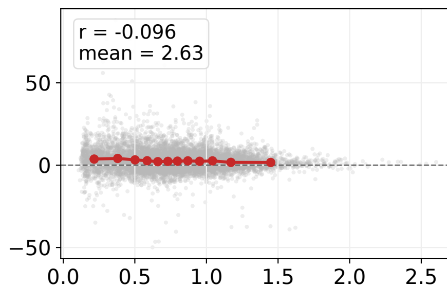
vs. FlowRefiner-PDE
