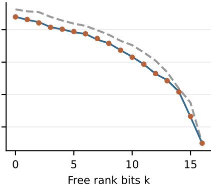
C T, m=20
