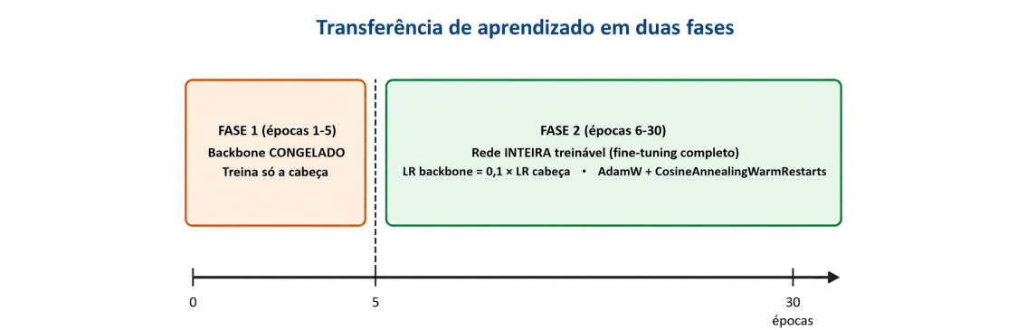
Figura 5. Fases da Transferência de aprendizado
