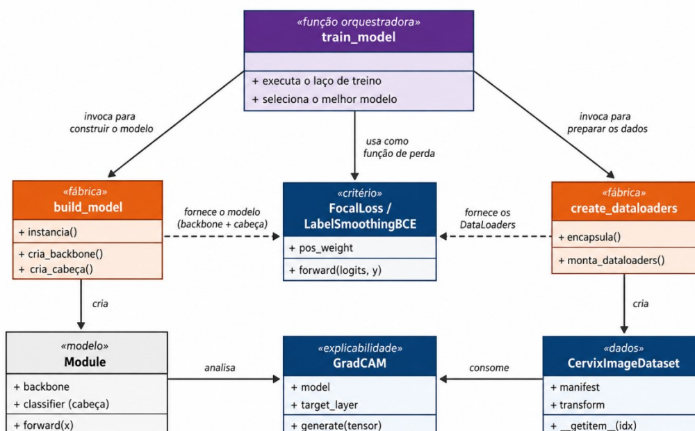
Diagrama UML de dependências: orquestração do treinamento
