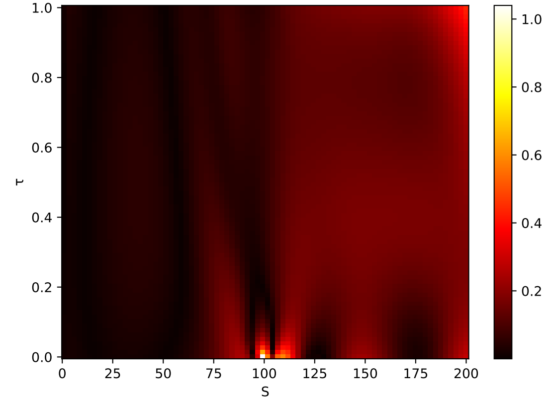
Absolute Error
