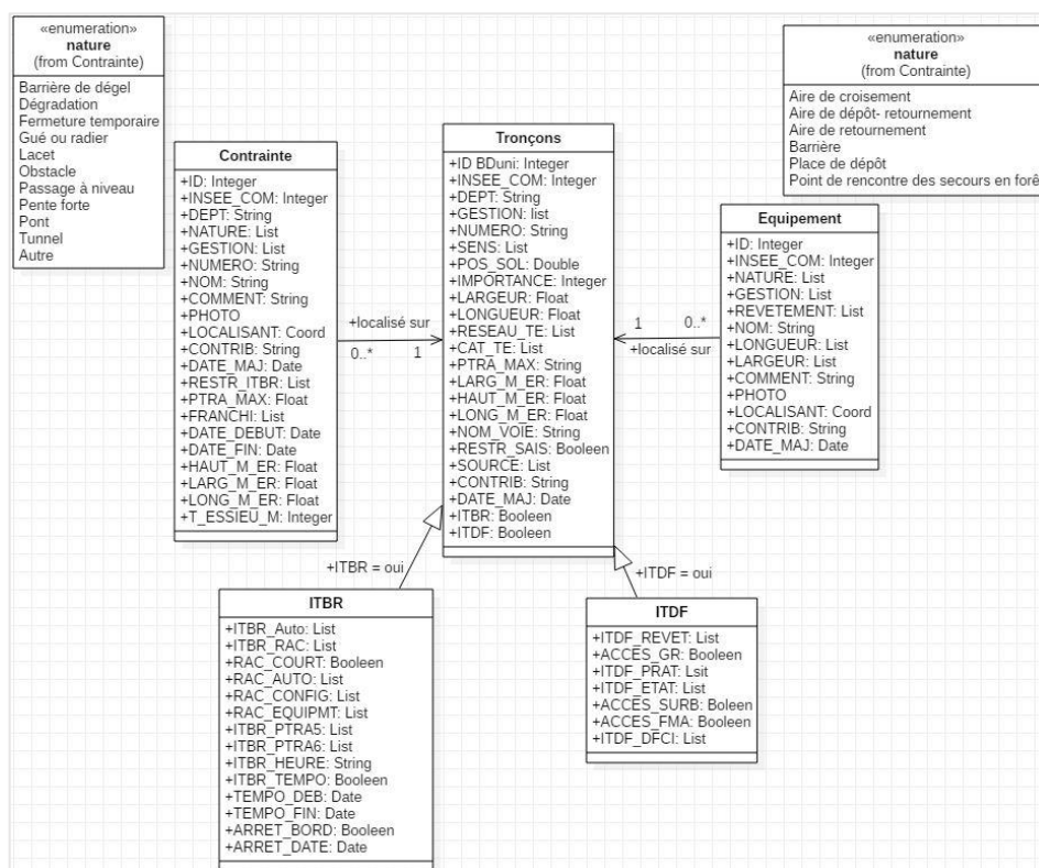
Figure 18: Modèle de données du standard national "desserte pour le transport de bois"
