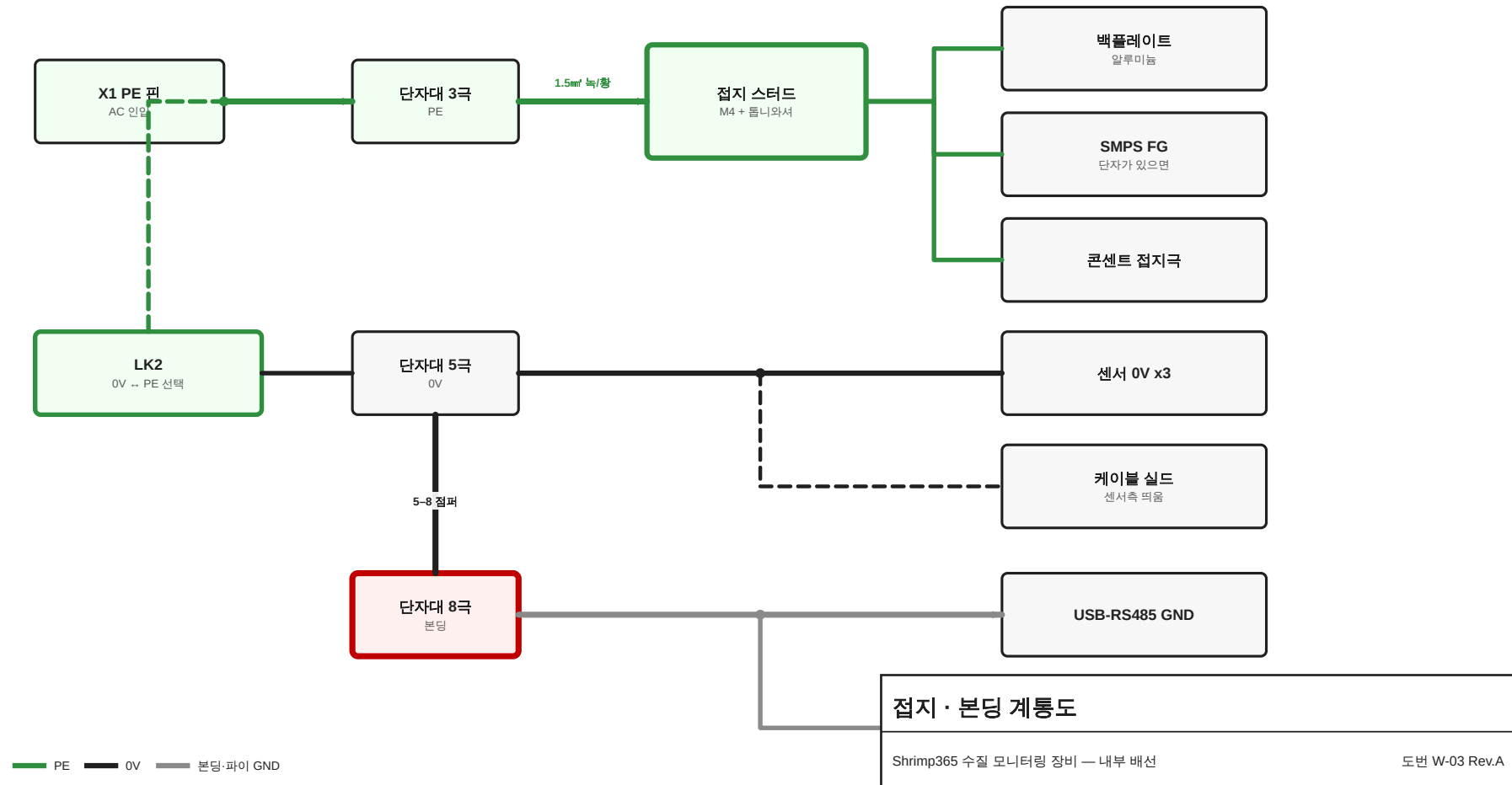
W-03 접지 · 본딩 계통도
