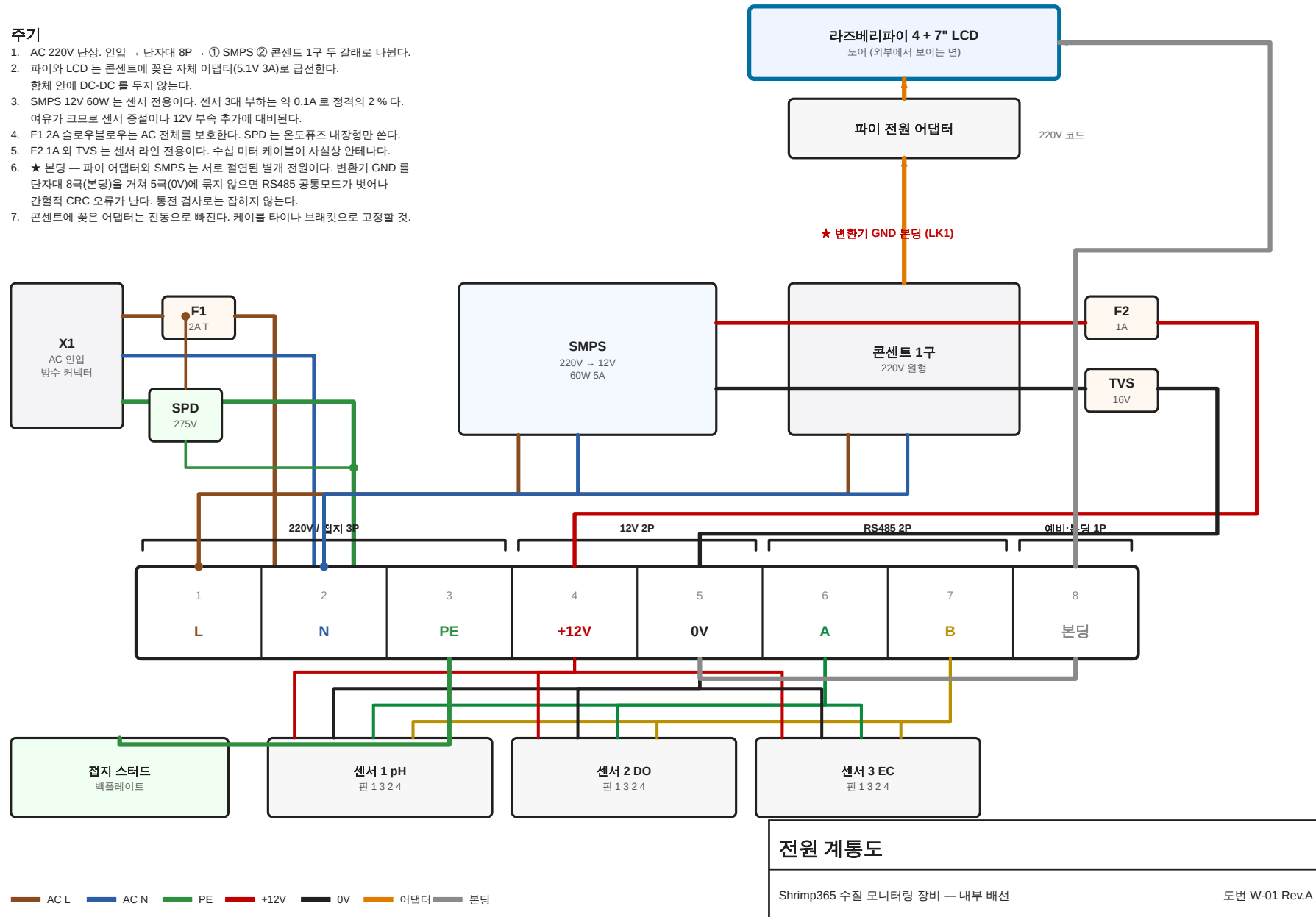
W-01 전원 계통도
