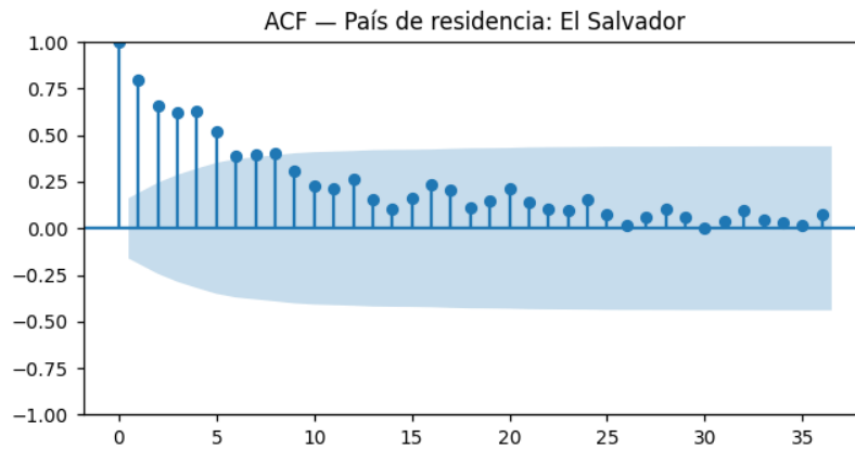
Figura. Función de autocorrelación (ACF, 36 rezagos).
