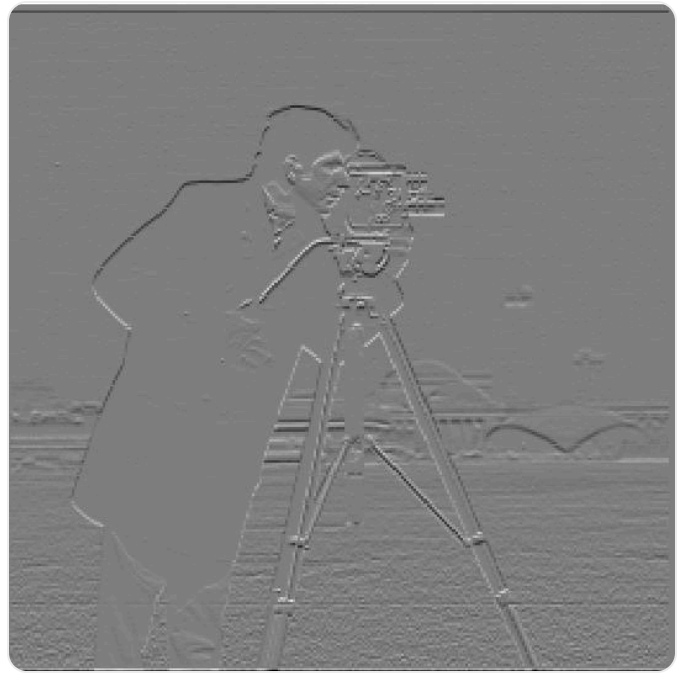
\partial/\partial Y
