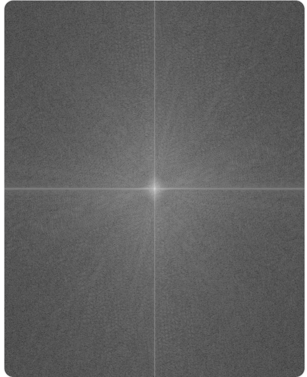
HYBRID · FFT
