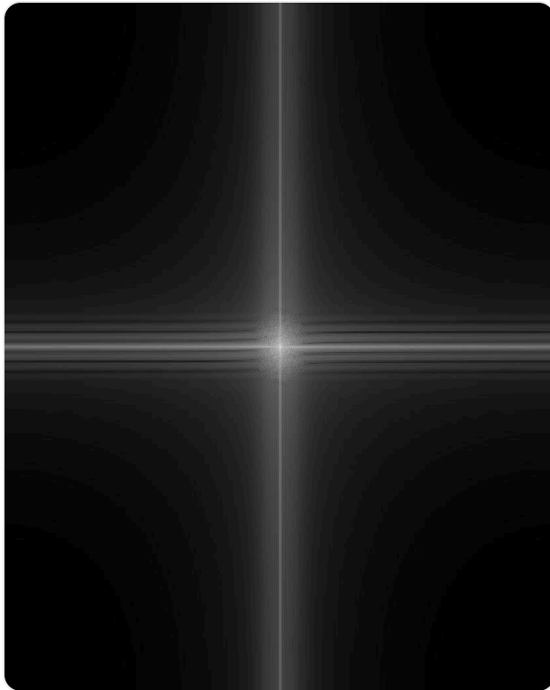
FFT · LOW-PASS
