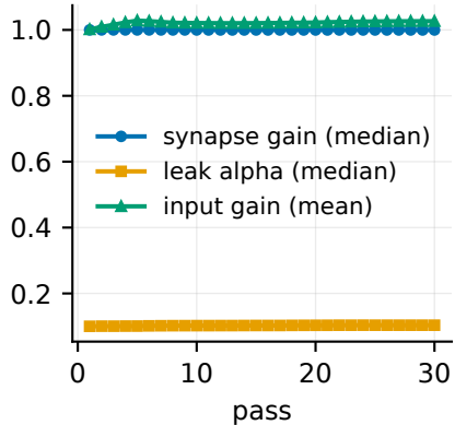
Brain parameters
