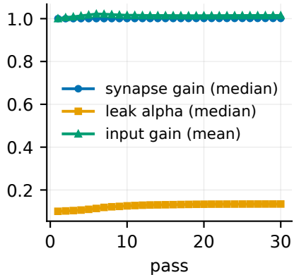
Brain parameters
