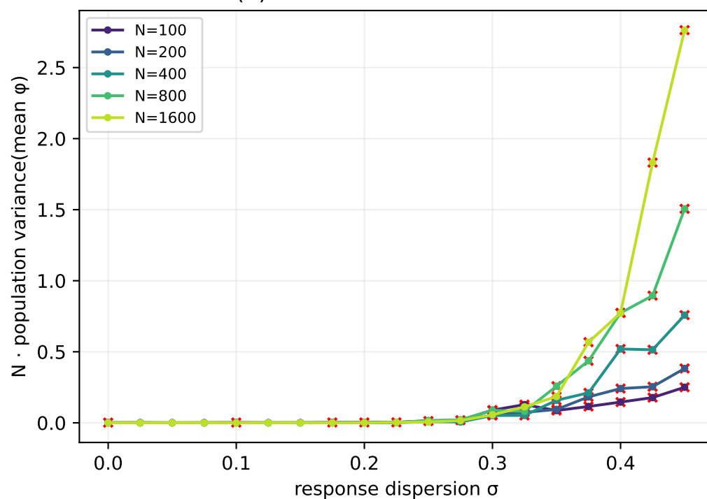
(d) Between-run fluctuations
