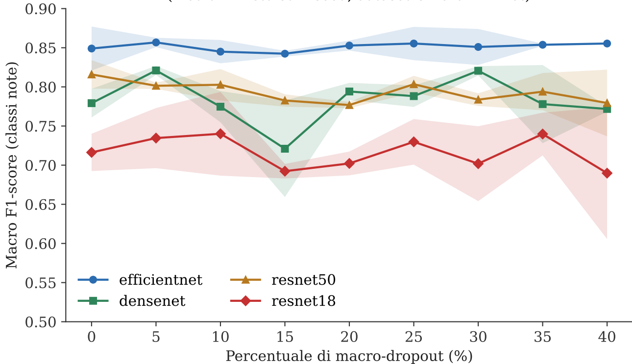
Andamento del Macro F1 al crescere del macro-dropout (media \pm 1 std su 2 seed, dataset Oxford-IIIT Pet)
