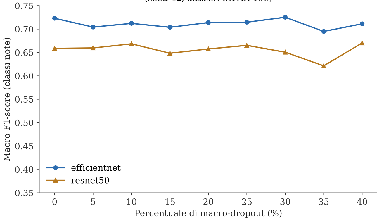
Andamento del Macro F1 al crescere del macro-dropout (seed 42, dataset CIFAR-100)
