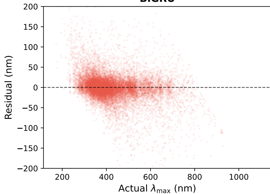
BiGRU
