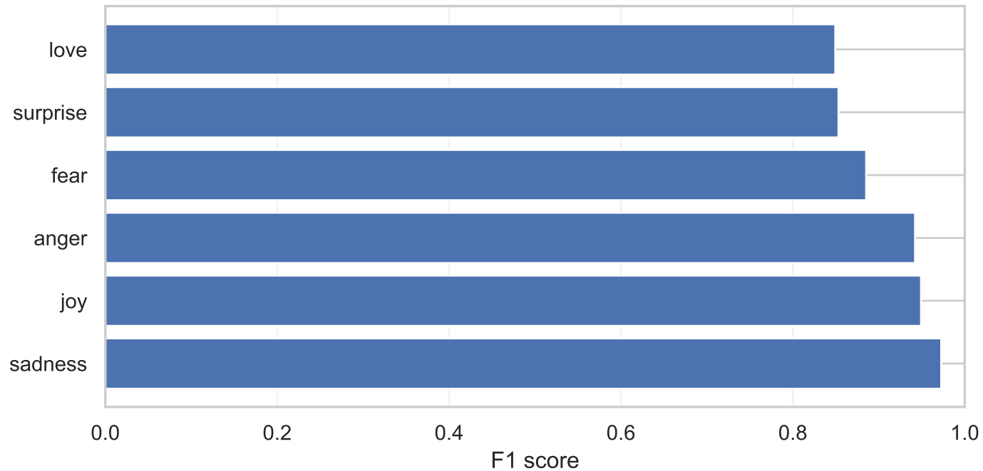
Emotion per-class F1
