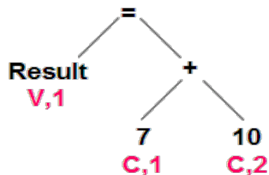
(a)一种具体的语句及其解析结构
