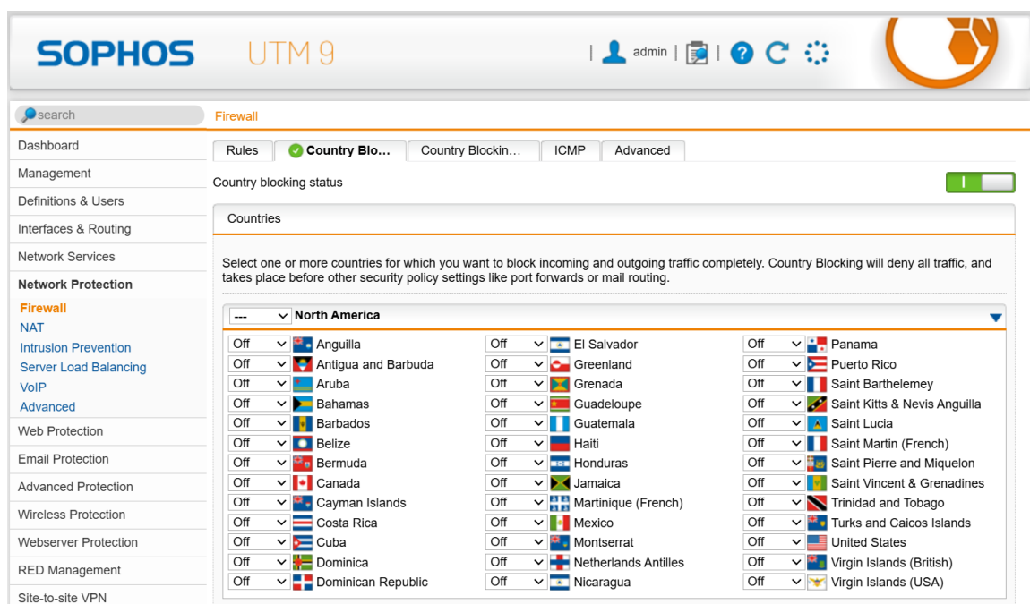
Hình 4. Vào Country Blocking để cấu hình các chính sách về quốc gia
