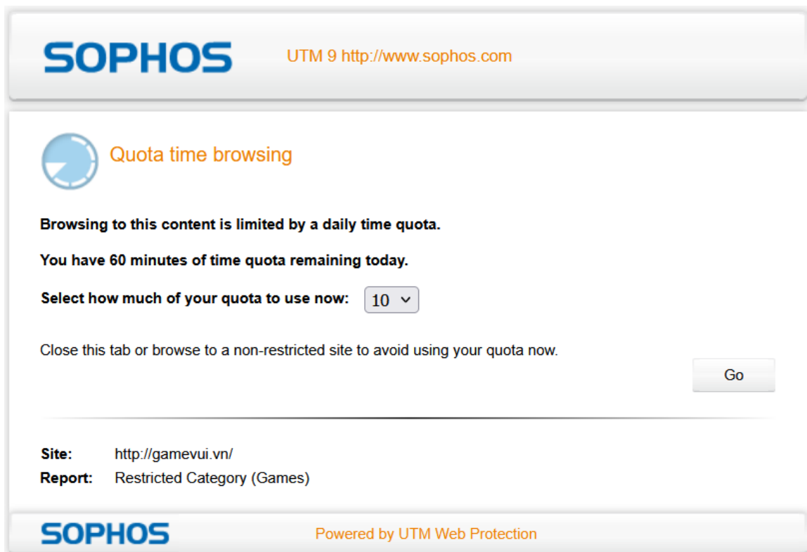
Hình 33. Kịch bản 5: Thời gian truy cập Gamevui.vn bị giới hạn 60 phút
