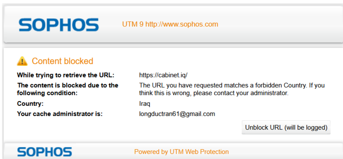
Hình 24. Kịch bản 2: Chặn truy cập vào các Website của quốc gia bị chặn (3)
