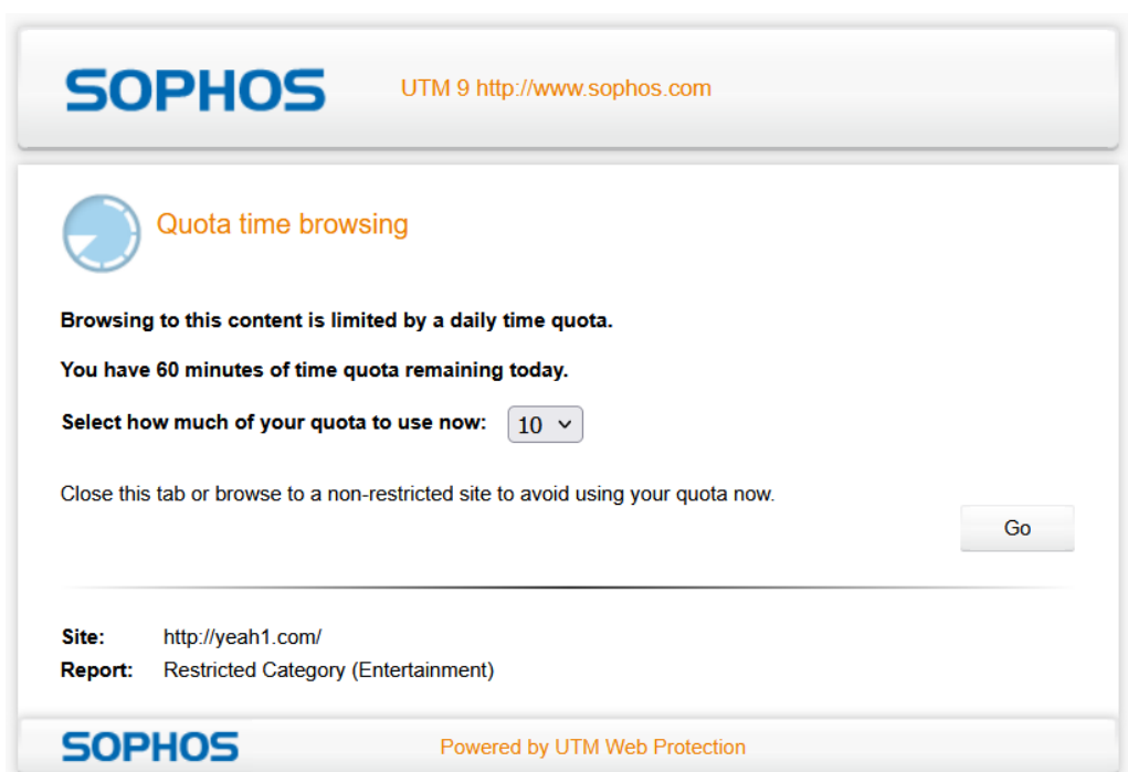
Hình 32. Kịch bản 5: Thời gian truy cập Yeah1.com bị giới hạn 60 phút
