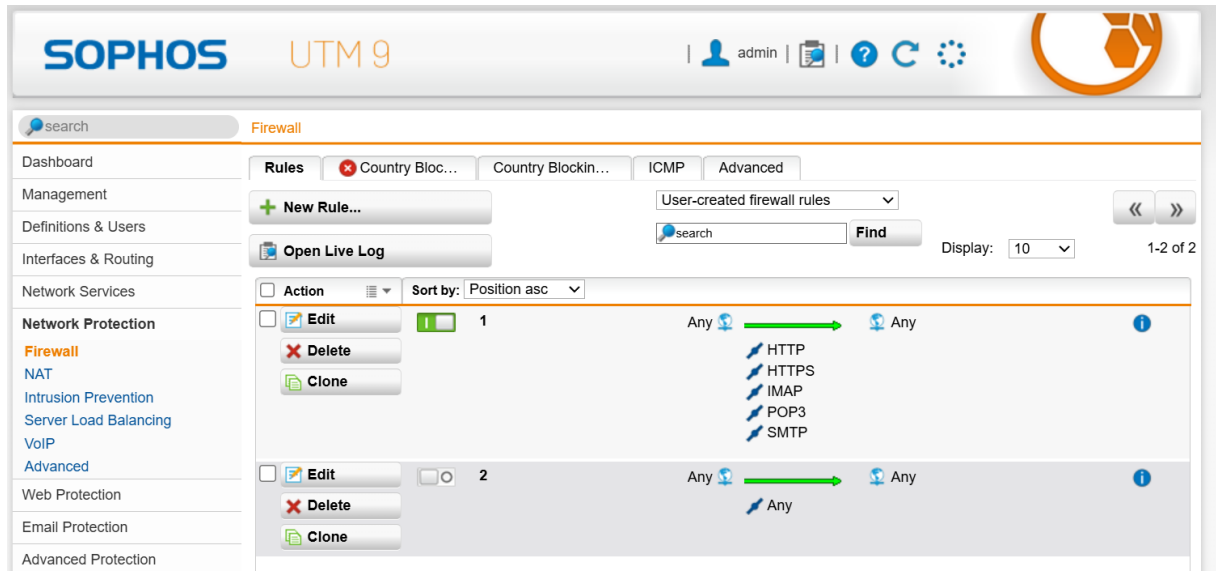
Hình 2. Cấu hình bộ lọc các giao thức có thể truy cập
