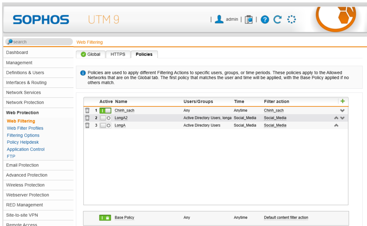
Hình 20. Cấu hình Policies và hoàn tất cấu hình
