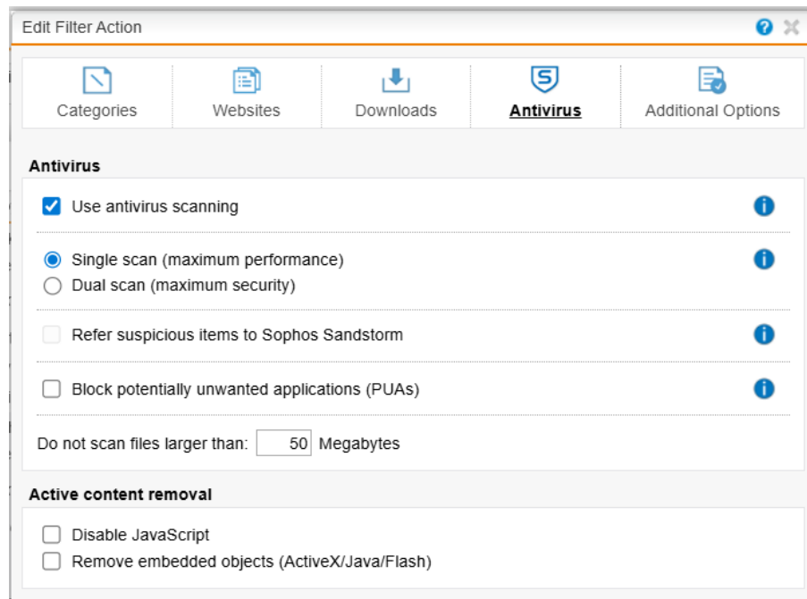
Hình 15. Cấu hình quét virus khi tải các tập tin
