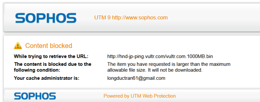
Hình 42. Kịch bản 7: File 1000MB bị chặn và không thể tải
