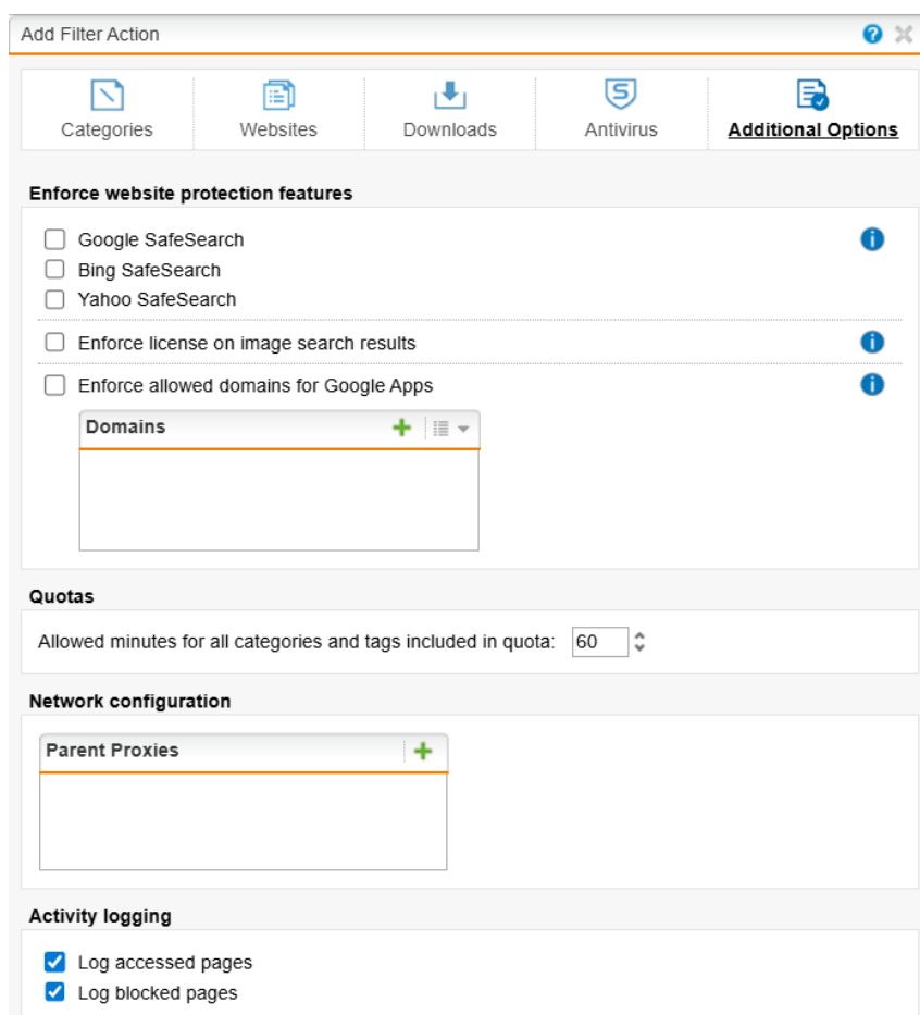
Hình 14. Cấu hình giới hạn thời gian sử dụng của các mục được chọn Quota
