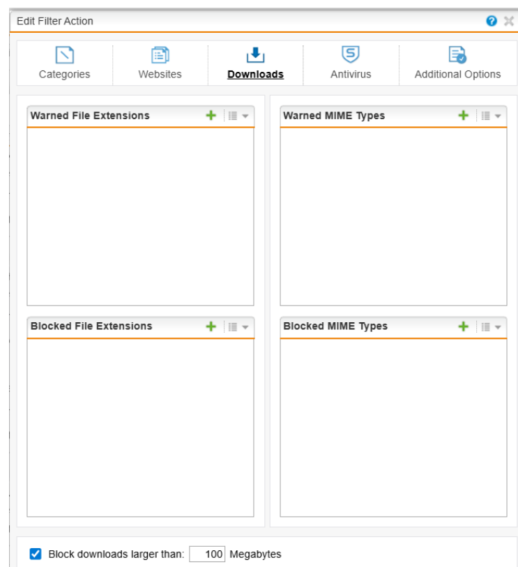
Hình 16. Cấu hình giới hạn dung lượng File khi tải
