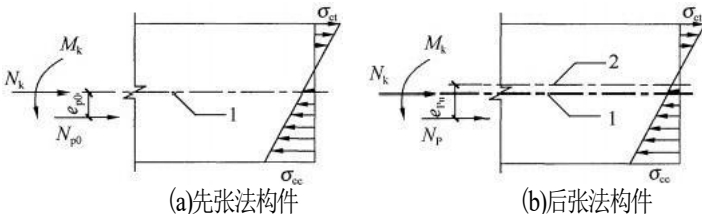
图10.1.11 预应力混凝土构件施工阶段验算
