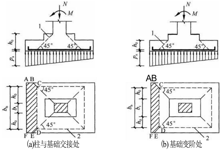
图6.5.5 计算阶形基础的受冲切承载力截面位置 1—冲切破坏锥体最不利一侧的斜截面; 2—冲切破坏锥体的底面线
