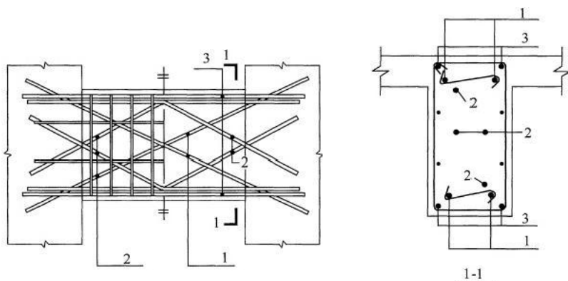
图11.7.10-1 交叉斜筋配筋连梁
