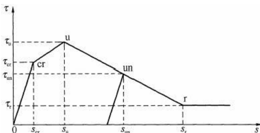
图C.3.1 混凝土与钢筋间的粘结应力-滑移曲线
