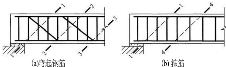
图6.3.2 斜截面受剪承载力剪力设计值的计算截面 1-1支座边缘处的斜截面; 2-2、3-3受拉区弯起钢筋弯起点的斜截面; 4-4箍筋截面面积或间距改变处的斜截面
