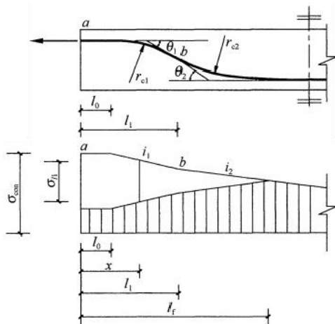
图J.0.3-2 两条圆弧形曲线组成的预应力筋的预应力损失 o
