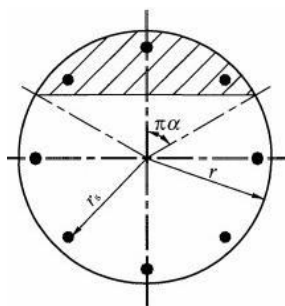
图 E.0.4 沿周边均匀配筋的圆形截面
