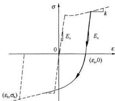
图C.1.3 钢筋反复加载应力-应变曲线
