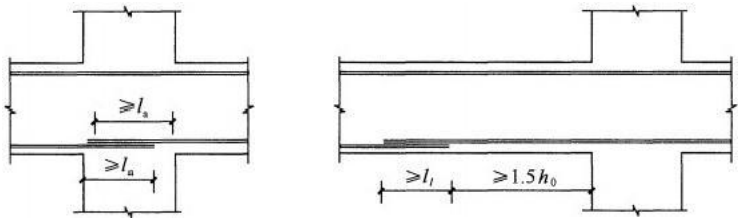
(a) 下部纵向钢筋在节点中直线锚固 (b) 下部纵向钢筋在节点或支座范围外的搭接
