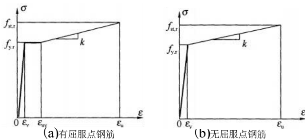
图C.1.2 钢筋单调受拉应力-应变曲线
