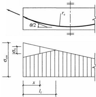
图J.0.3-1 圆弧形曲线预应力筋的预应力损失 \sigma
