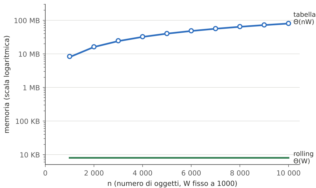
Figura 3: Occupazione di memoria della tabella, calcolata dalla formula (linea) e misurata sull'heap (cerchi), a confronto con quella della variante a spazio ridotto, di cui si riporta la sola formula (Sezione 7.1).
