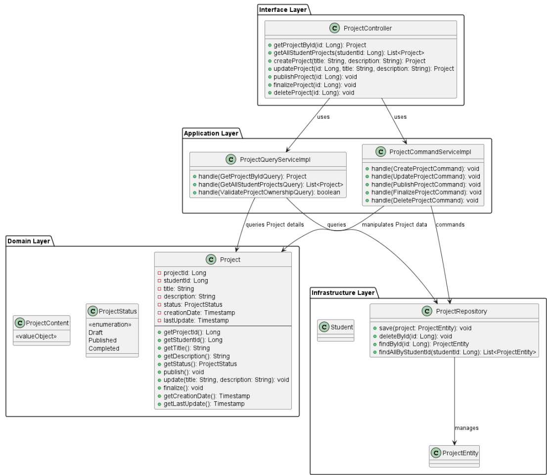
Bounded Context Class Diagram - Elaboración propia
