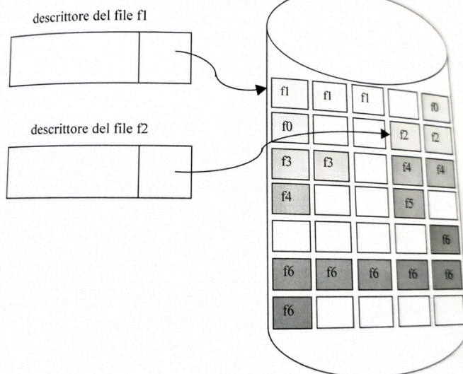
Figura 6.7 Allocazione contigua di file.
