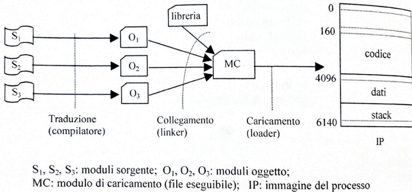
Figura 4.2 Preparazione di un programma per l'esecuzione.
