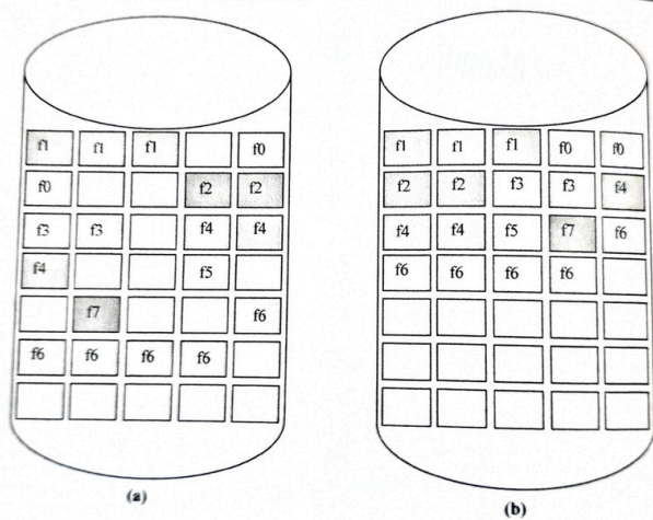
Figura 6.8 Frammentazione dello spazio disponibile su disco (a) e compattamento (b).
