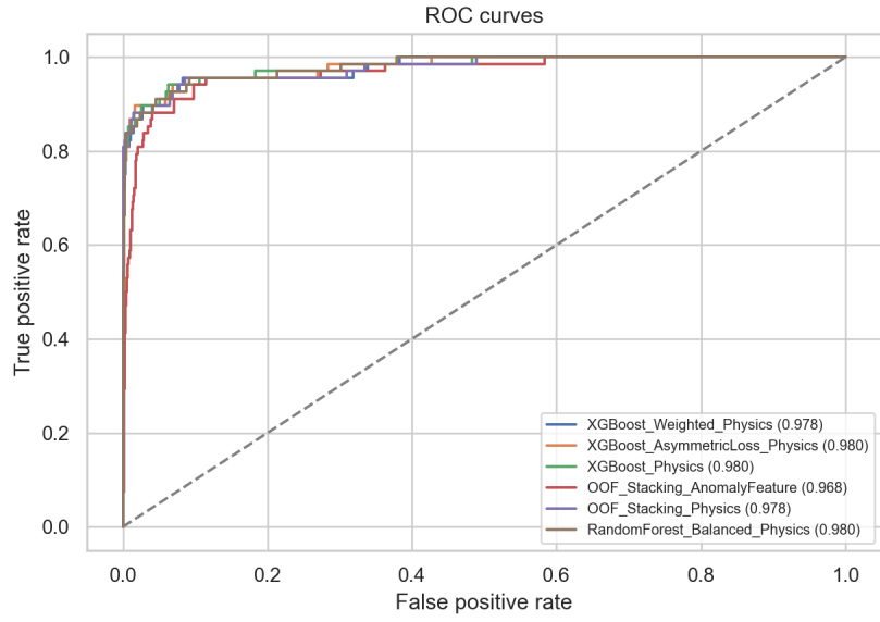
图 5.5: ROC 曲线
