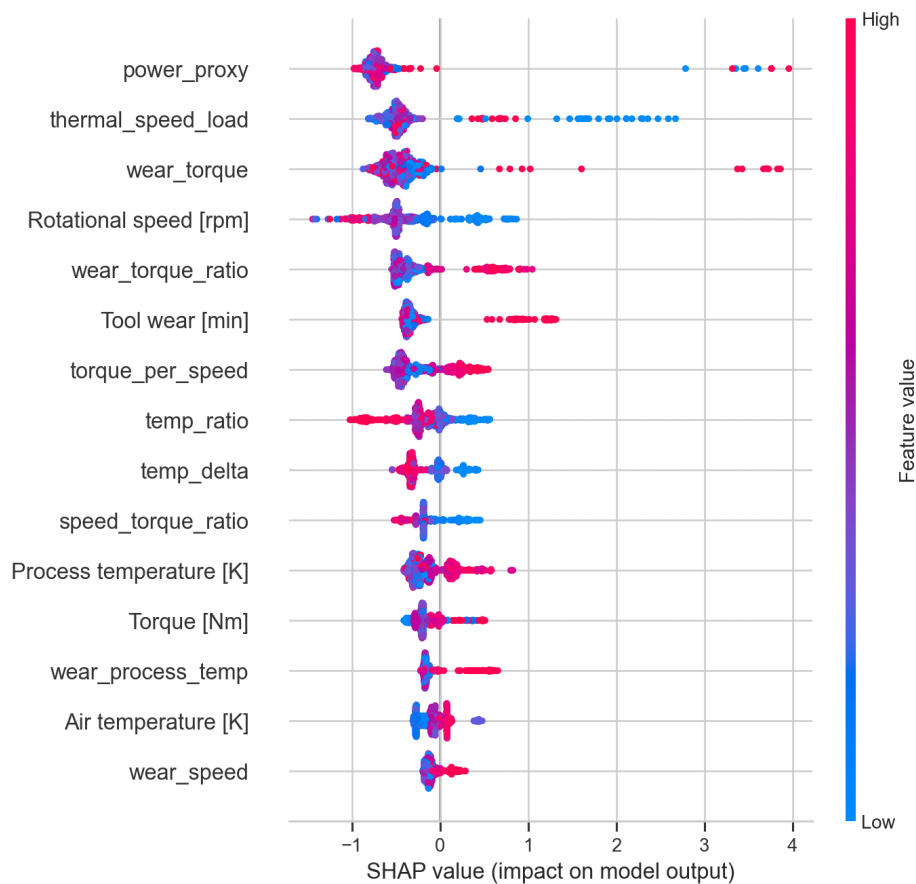
图 6.2: SHAP 分析
