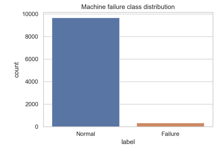
图 2.1: 类别分布
