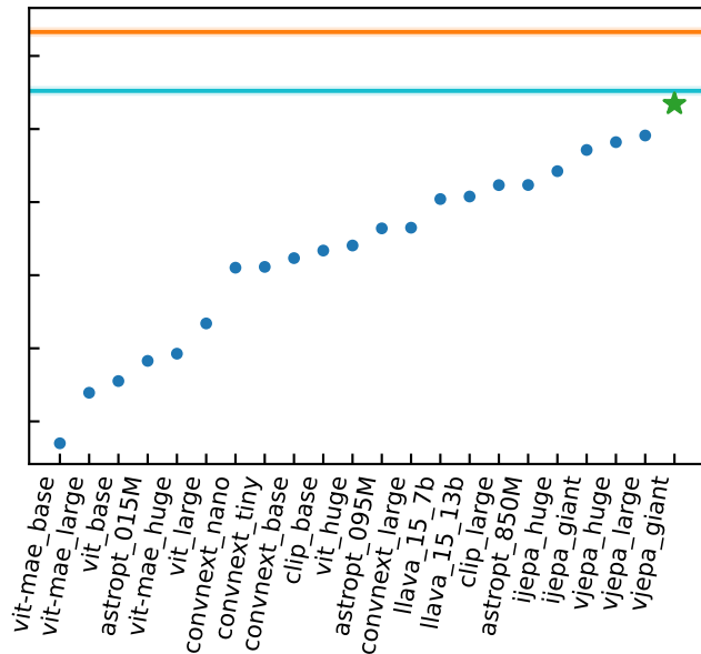
JWST
