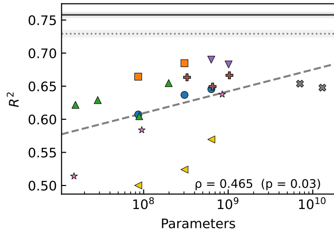
redshift ( R^2 )
