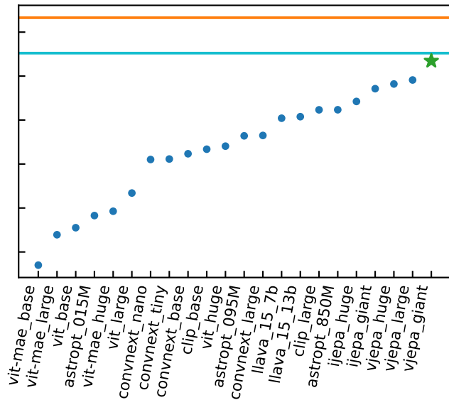
JWST
