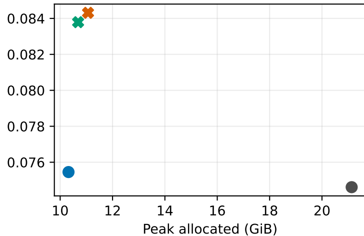
BONN
