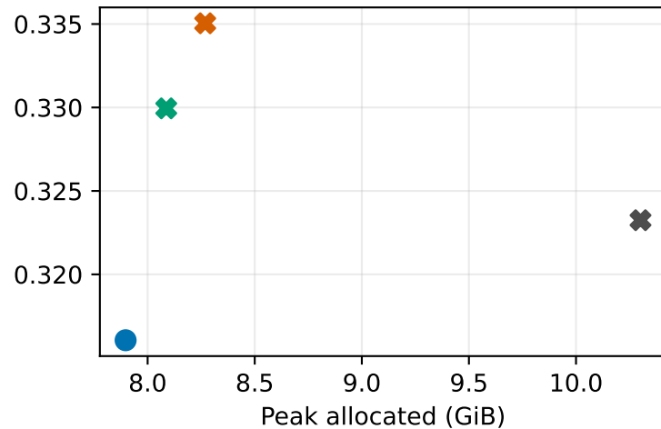
SINTEL
