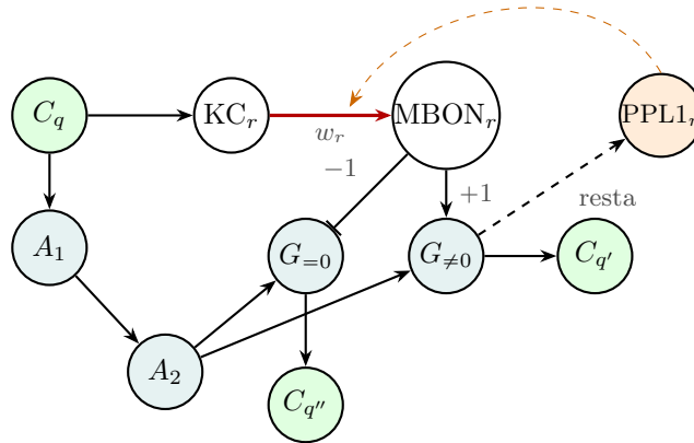
FIGURA 4. El circuito que ejecuta una pregunta ?r \leadsto (A) \mid (B) . La neurona del paso ( C_q ) enciende la KC, que lee la variable: la MBON solo responde si la variable no es cero. A la vez, la señal pasa por dos neuronas de retardo ( A_1, A_2 ) para llegar a las dos compuertas justo cuando llega la respuesta de la MBON. Si la MBON respondió, se enciende la compuerta de arriba, que resta 1 mediante la PPL1 y pasa el turno al paso A ( C_{q'} ); si no, se enciende la de abajo y pasa el turno al paso B ( C_{q''} ). Las compuertas y los retardos (en turquesa) son neuronas locales del cuerno lateral.
