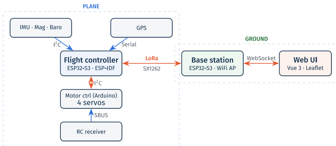
Abbildung 1: Systemtopologie: Flugzeug (Flugcontroller, IMU, GPS, Motoransteuerung, RC-Empfänger) verbunden per LoRa mit der Bodenstation, die per WebSocket mit der Web-UI kommuniziert
