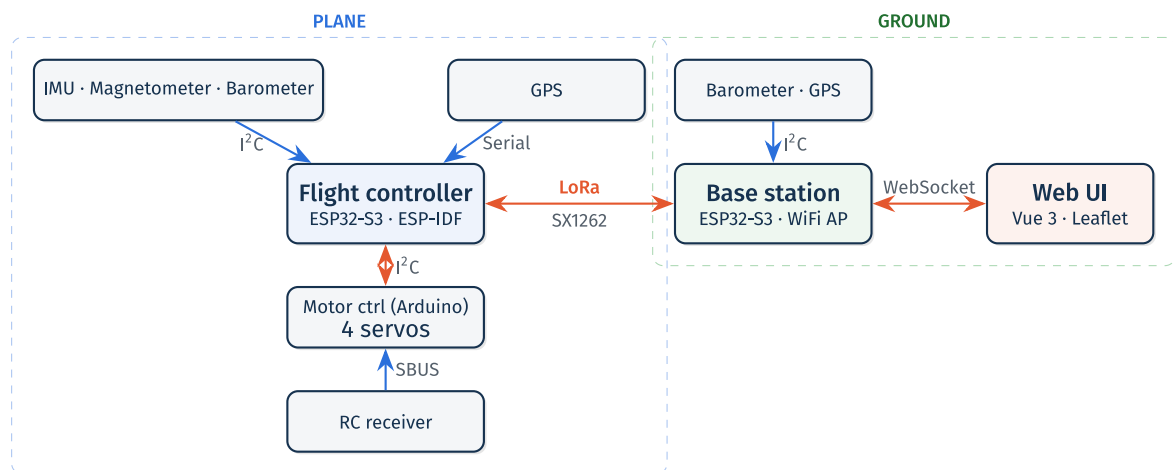
Abbildung 5: Systemtopologie: Flugzeug (Flugcontroller, IMU, GPS, Motoransteuerung, RC-Empfänger) verbunden per LoRa mit der Bodenstation, die per WebSocket mit der Web-UI kommuniziert
