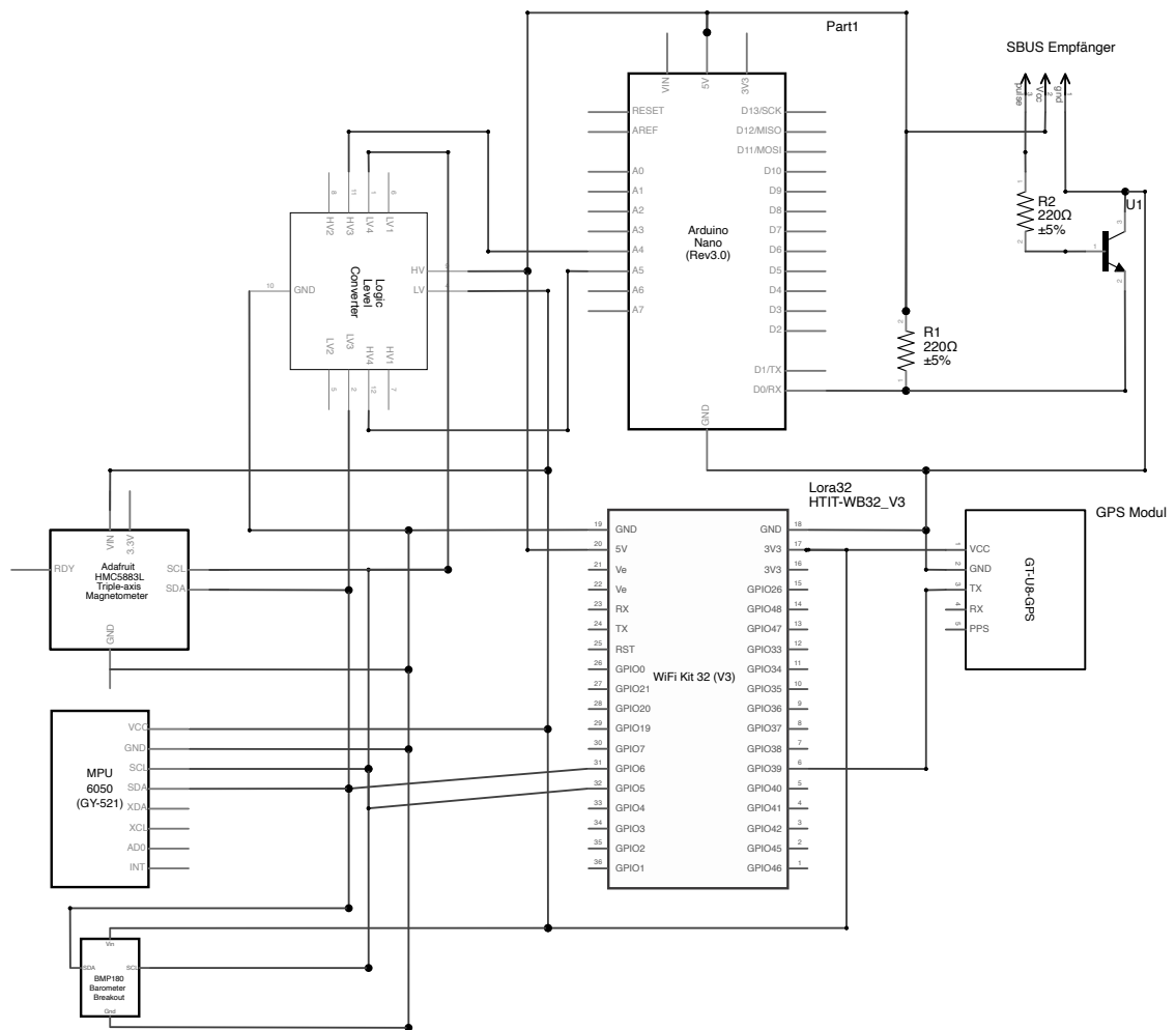
Abbildung 1: Schaltplan des Flugzeugs mit Heltec LoRa32 V3, GPS, IMU, Magnetometer, Barometer und Anbindung an den Arduino-Motor-Controller
