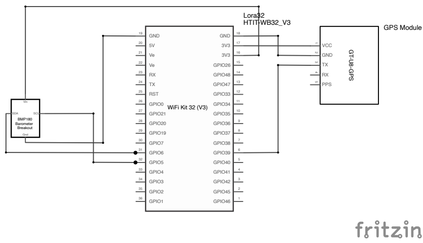
Abbildung 3: Schaltplan der Bodenstation mit Heltec LoRa32 V3, GPS und Barometer
