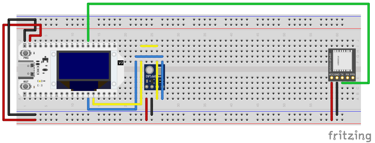
Abbildung 4: Steckplatten-Ansicht der Verkabelung der Bodenstation
