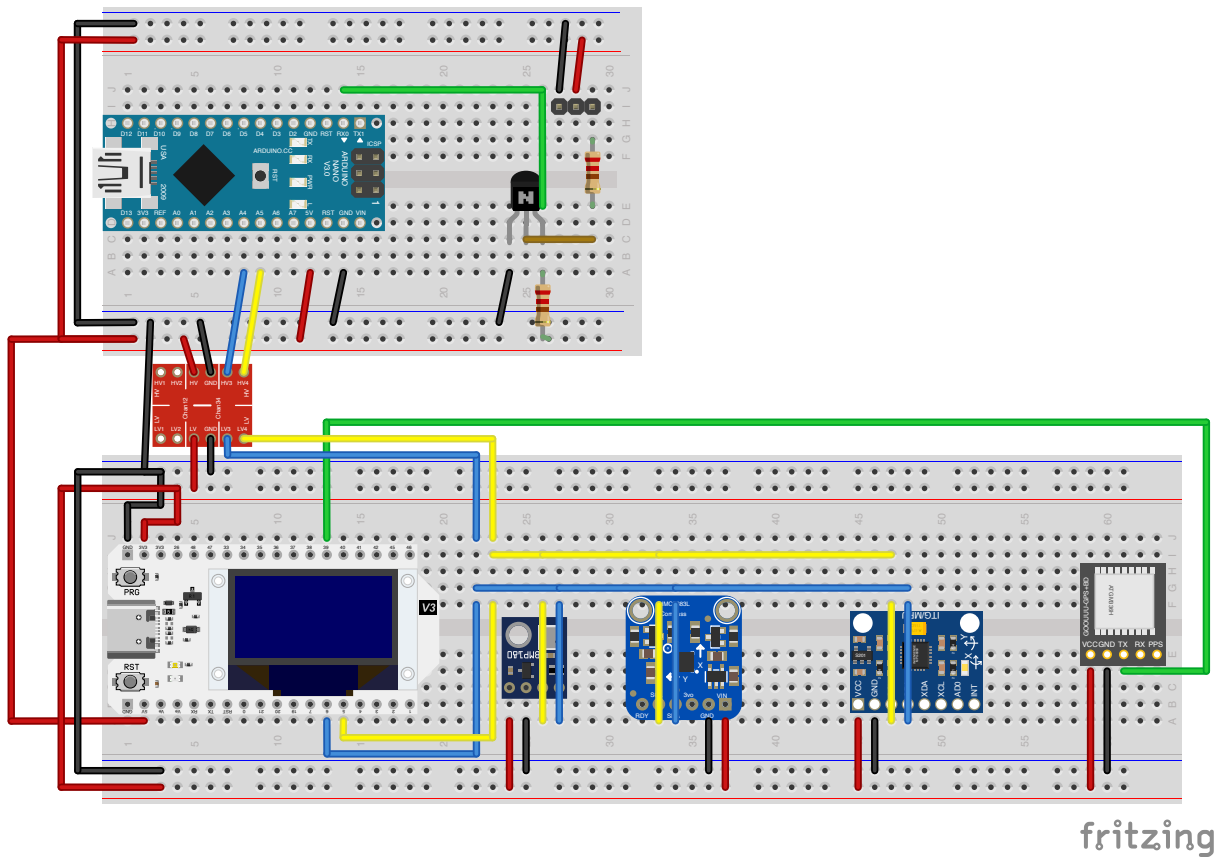
Abbildung 2: Steckplatten-Ansicht der Verkabelung im Flugzeug
