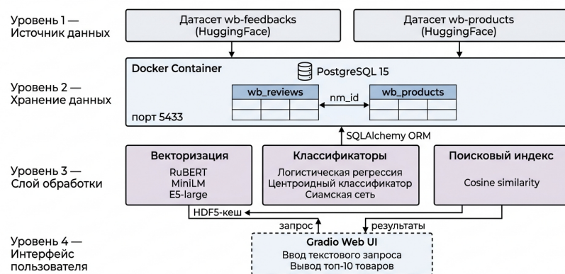
Рисунок 7 – Схема архитектуры рекомендательной системы
