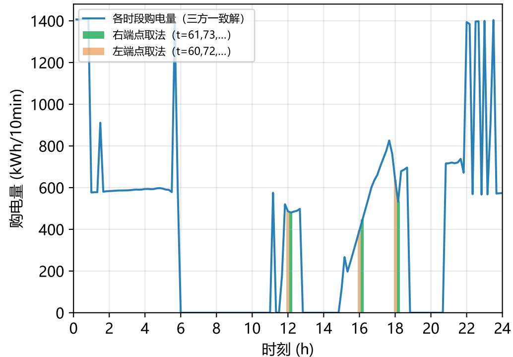
全天购电量曲线与两种取点位置
