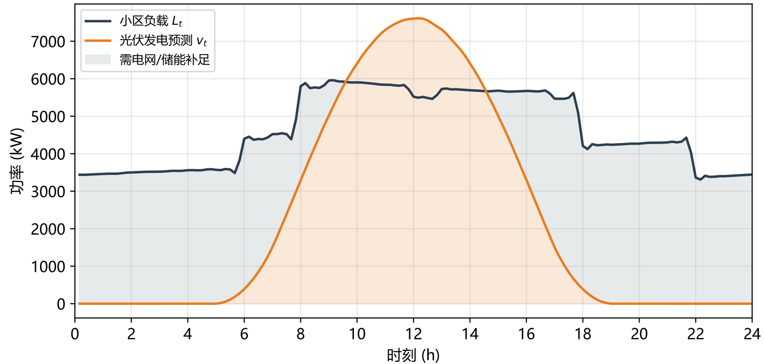
图2 小区负载与光伏发电预测功率
