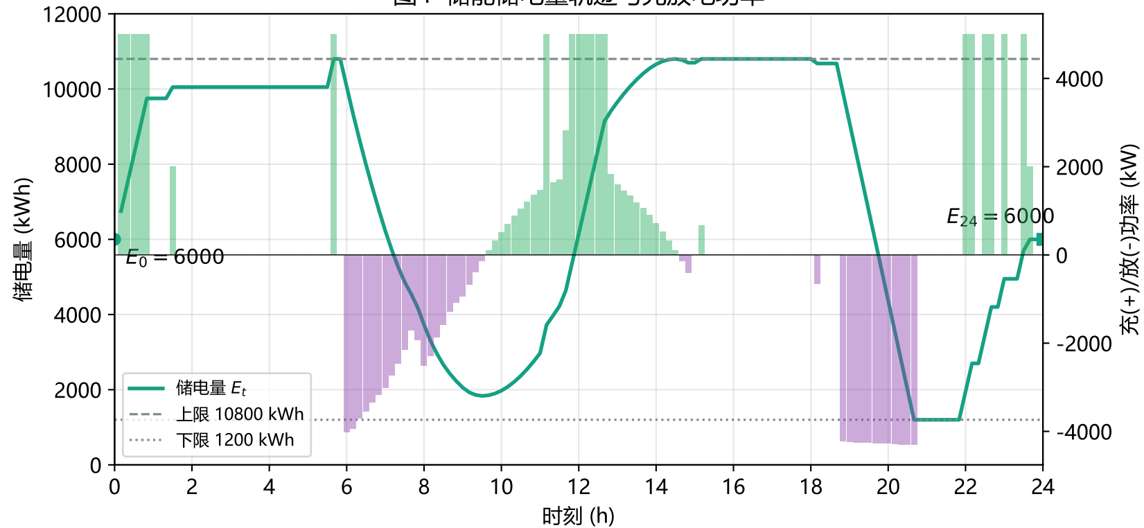
图4 储能储电量轨迹与充放电功率
