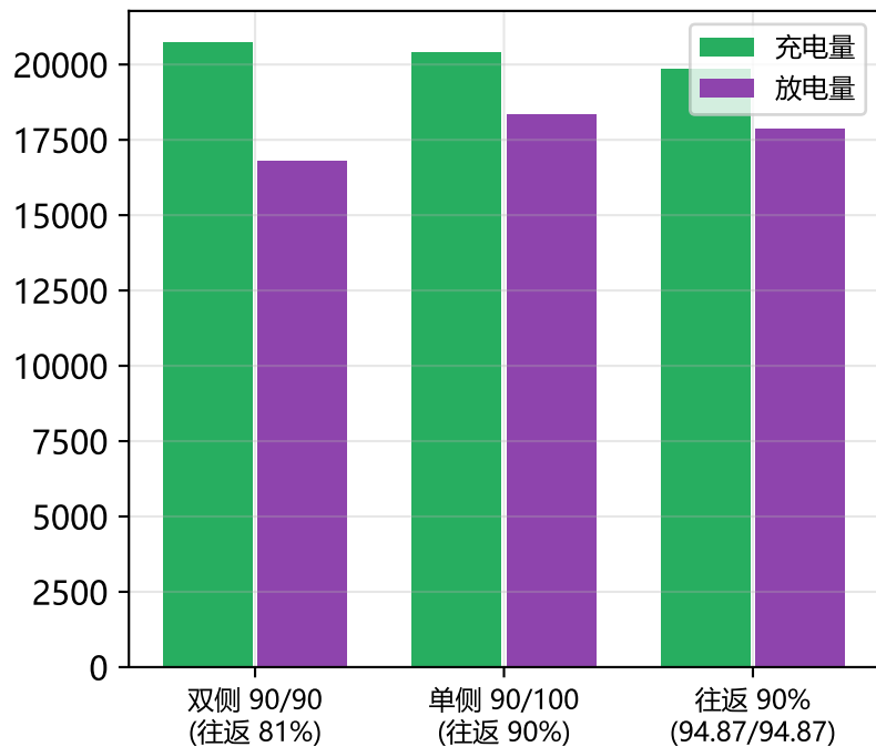
效率口径对充放电量的影响
