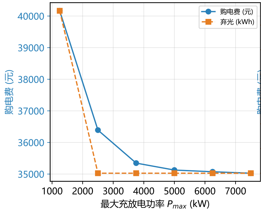
储能功率的影响
