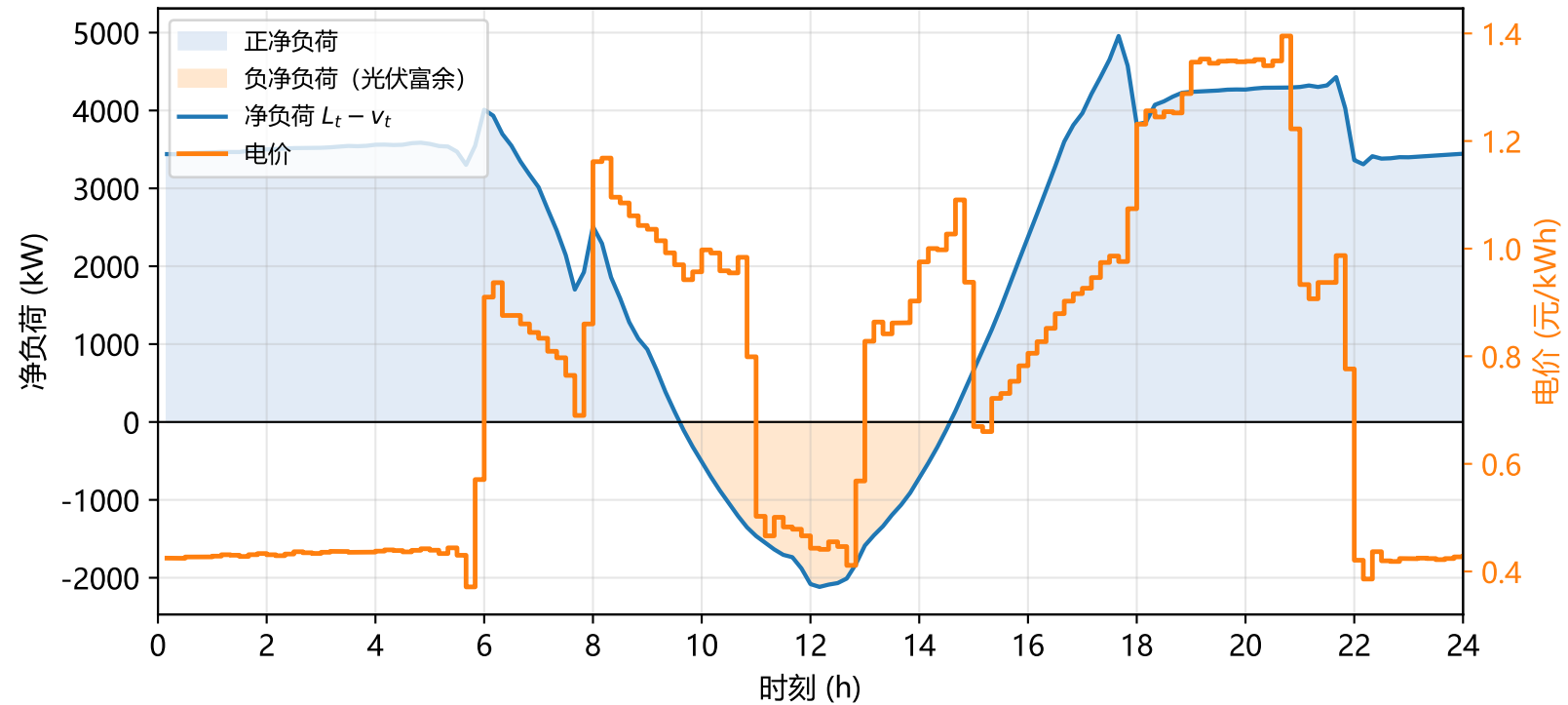
图1 全天电价与净负荷曲线 (附件1)
