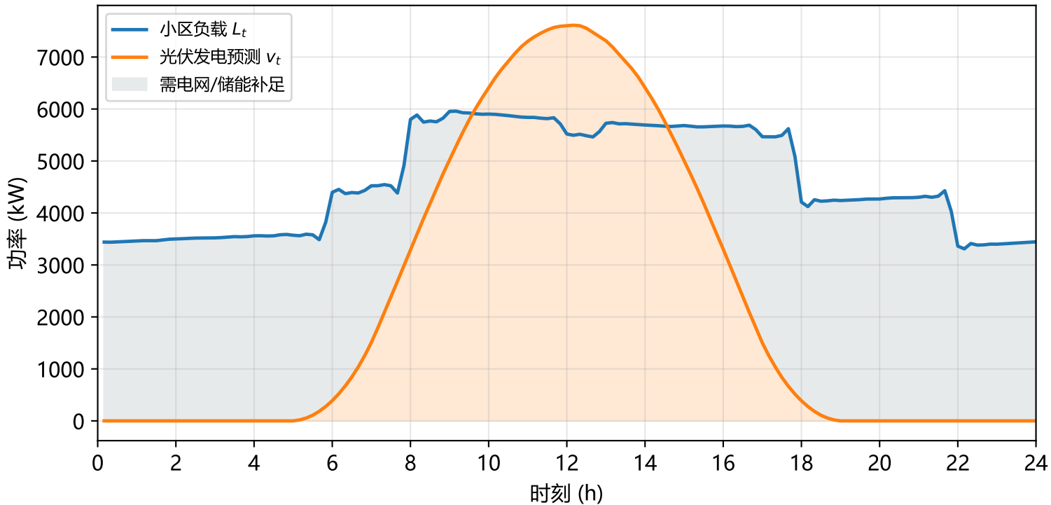
图2 小区负载与光伏发电预测功率
