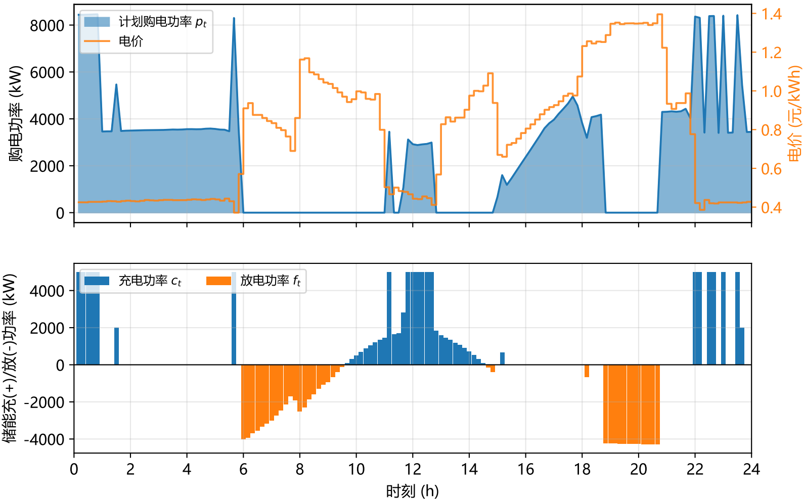
图3 最优计划购电策略 (GLM 路线: PuLP+CBC)
