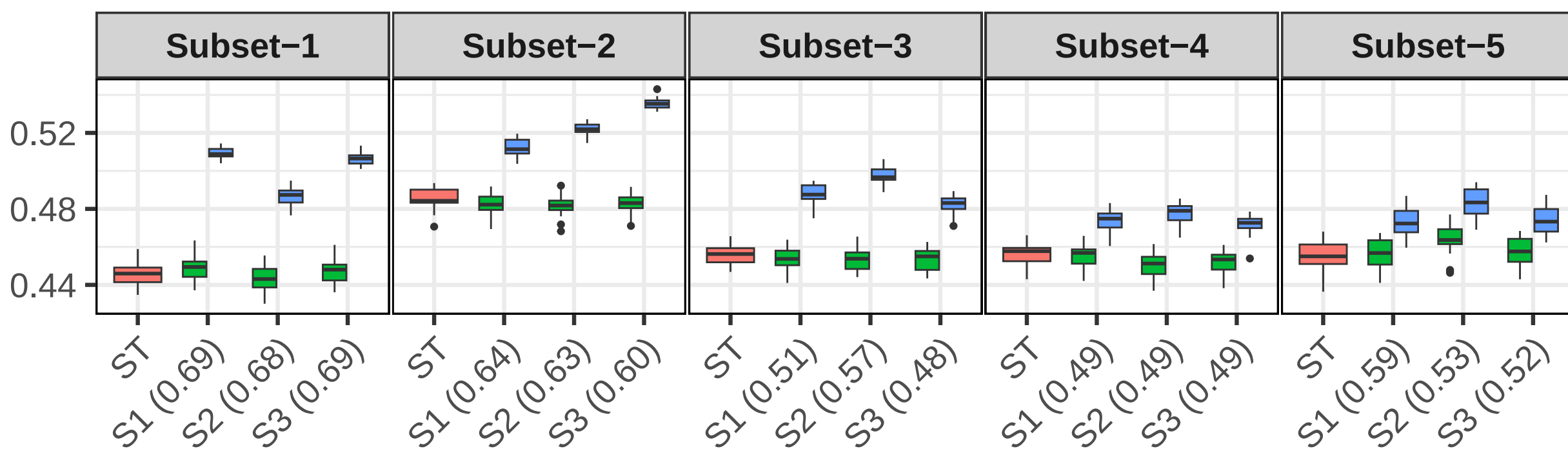
d PLSR-SLA
