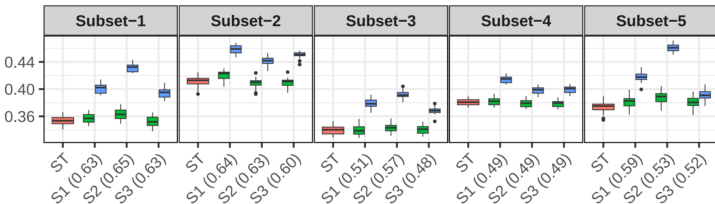
c PLSR-Narea
