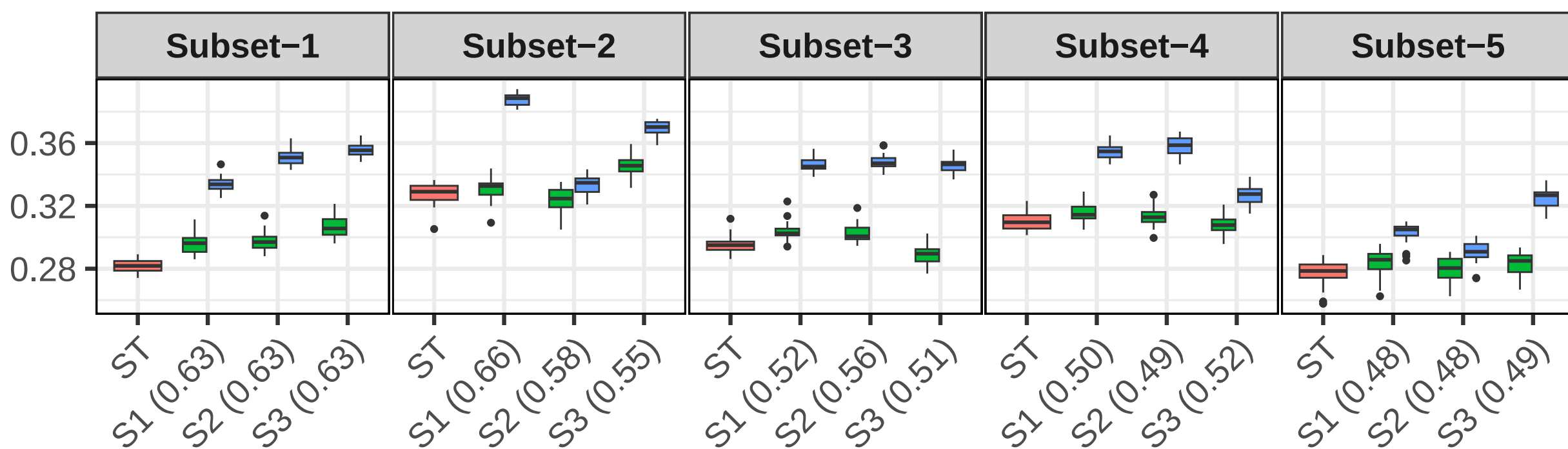
b SLA
