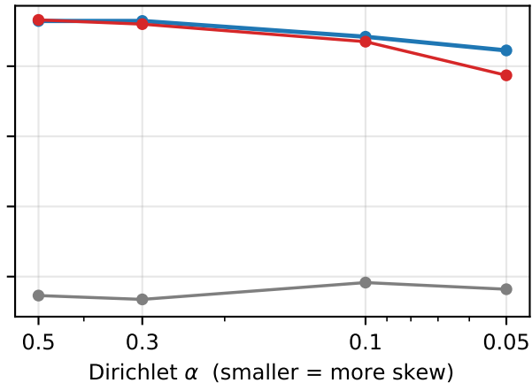
OrganAMNIST
