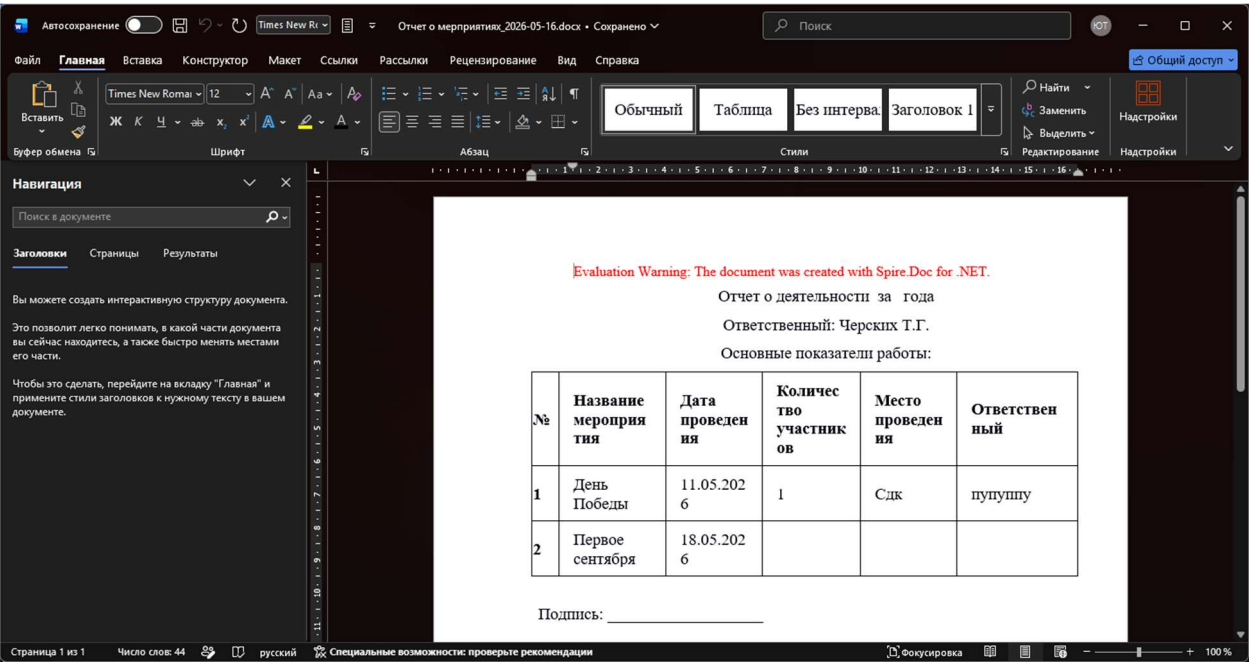
Рисунок 20 – Готовый отчет
