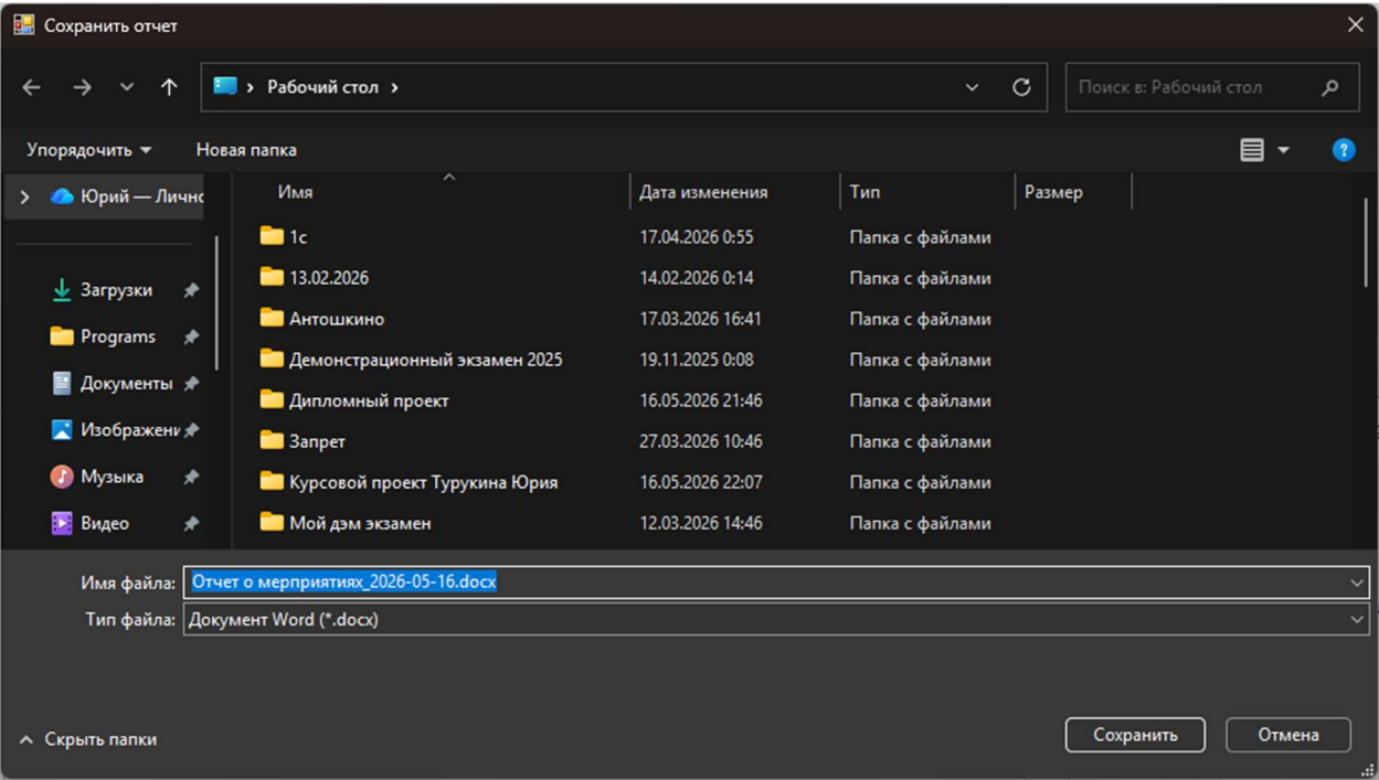
Рисунок 19 – Сохранение файла
