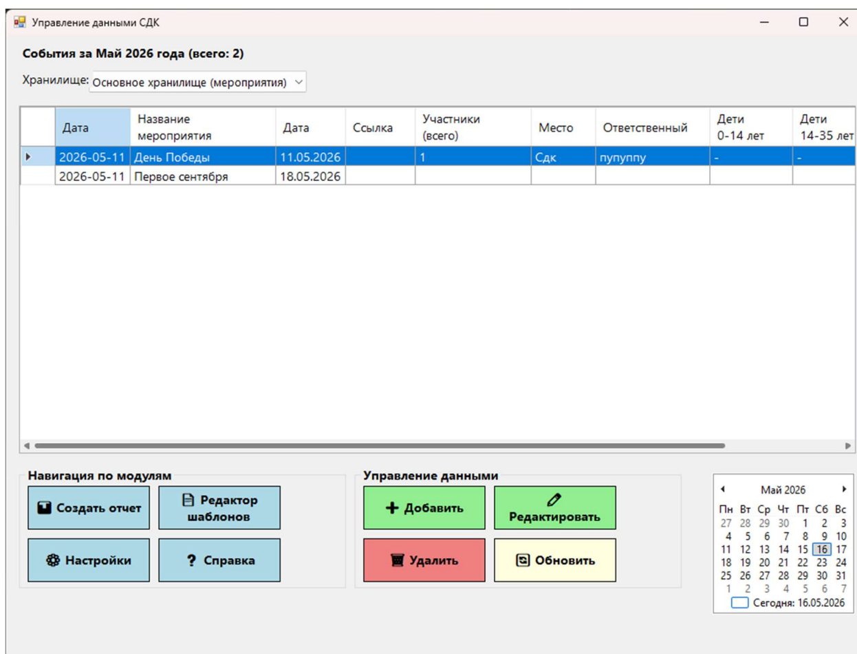
Рисунок 1 – Главная форма
