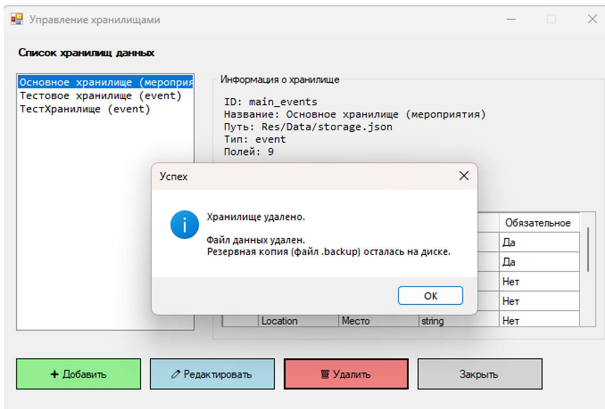
Рисунок 16 – Результат удаления
