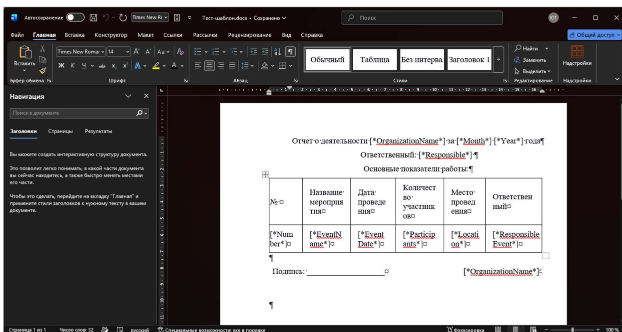
Рисунок 21 – Готовая заготовка.
