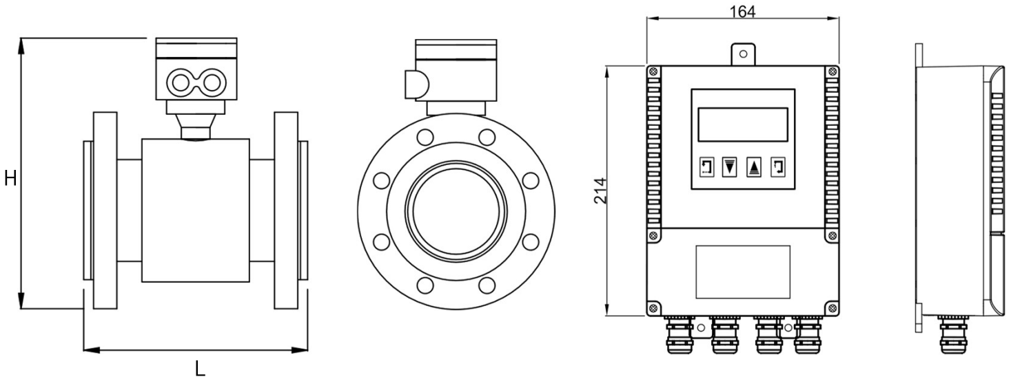
< Remote Type > 지시부 분리형 KM-200R
