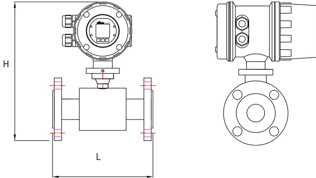
< Compact Type > 지시부 일체형 KM-200C
