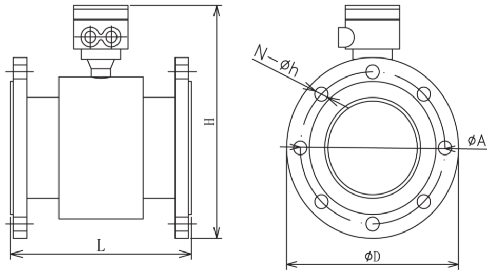
디스플레이 분리형 DIMENSION FOR REMOTE TYPE BODY
