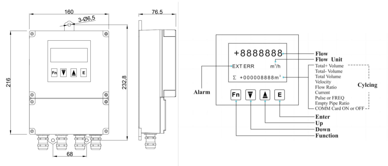
분리형 변환기 DIMENSION FOR REMOTE TYPE CONVERTER
