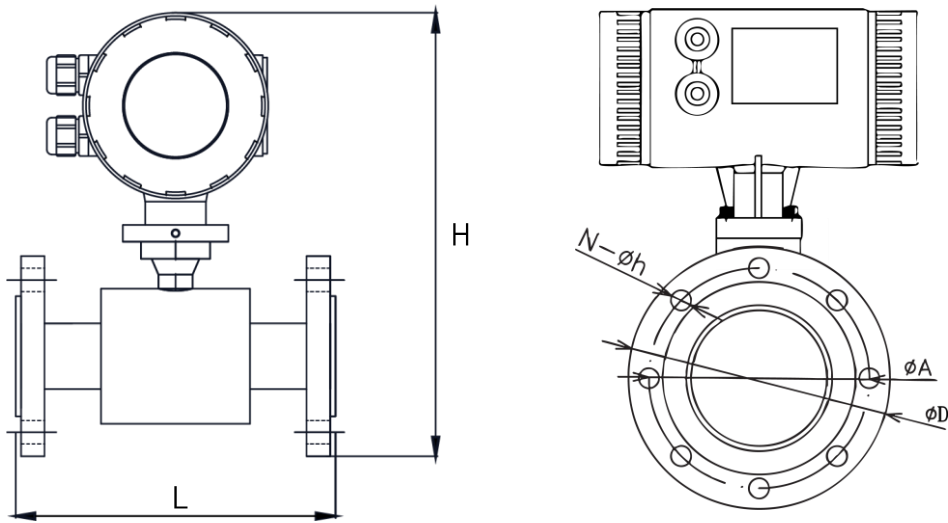
디스플레이 일체형 DIMENSION FOR COMPACT TYPE BODY
