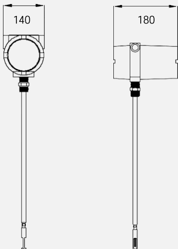
< Insertion Type > 삽입 일체형 KTM-8800
