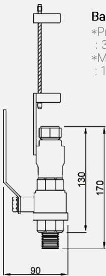
< Insertion Type Accessory > 삽입 분리형 부품 KTM-8200
