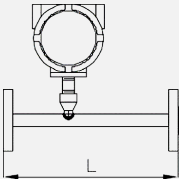
< Inline Type > 단관 일체형 KTM-8800
