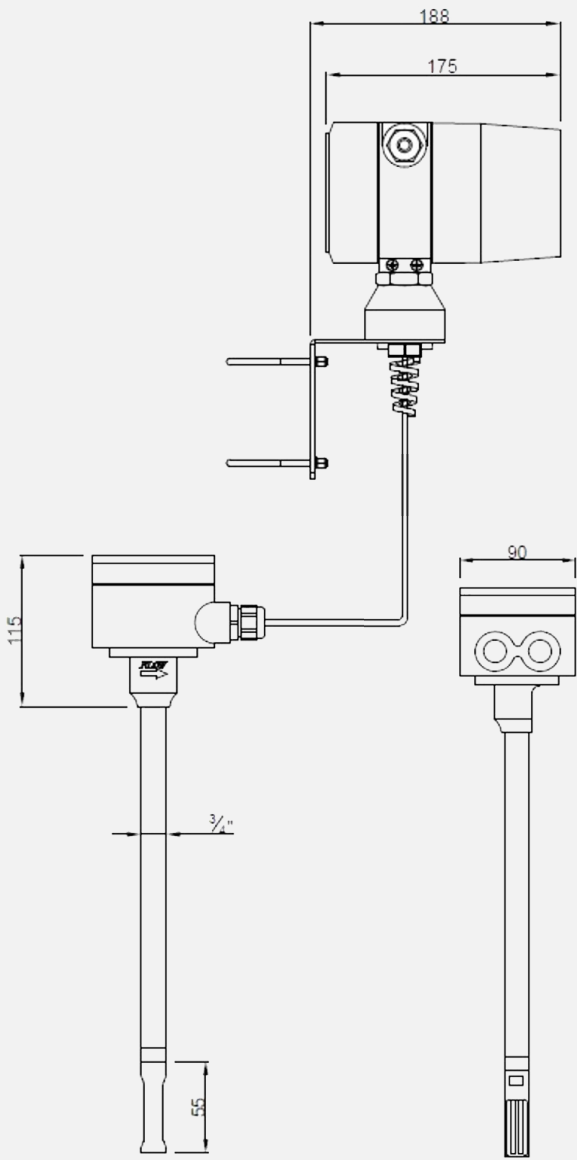
< Insertion Type > 삽입 분리형 검출부 KTM-8200
