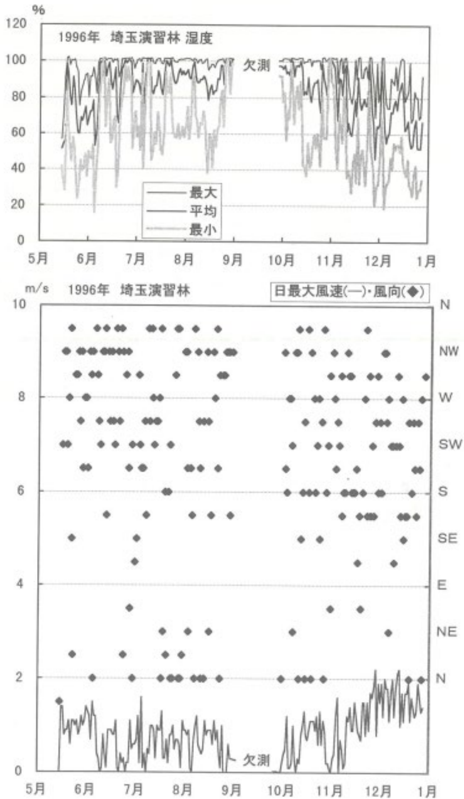
図3 埼玉演習林の湿度・風速・風向 (1996年5月～12月)
