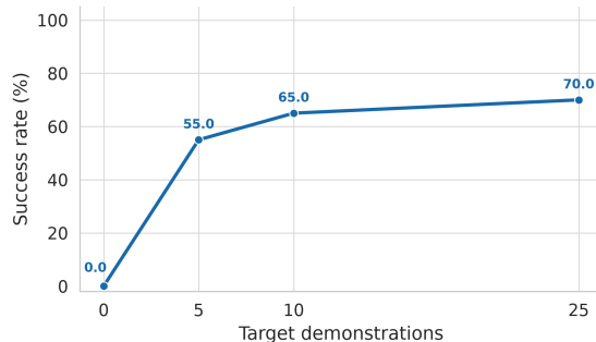
Рис. 1: Baseline success rate в зависимости от числа target-демонстраций
