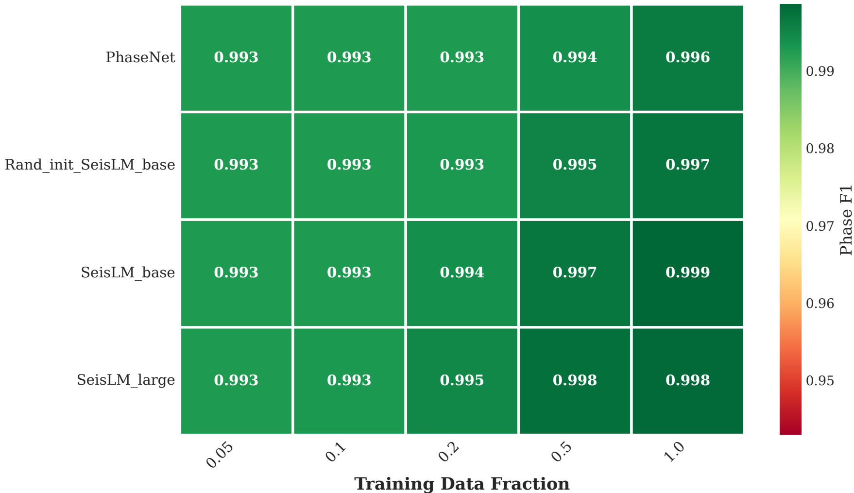
Phase Identification F1 Score - GEOFON
