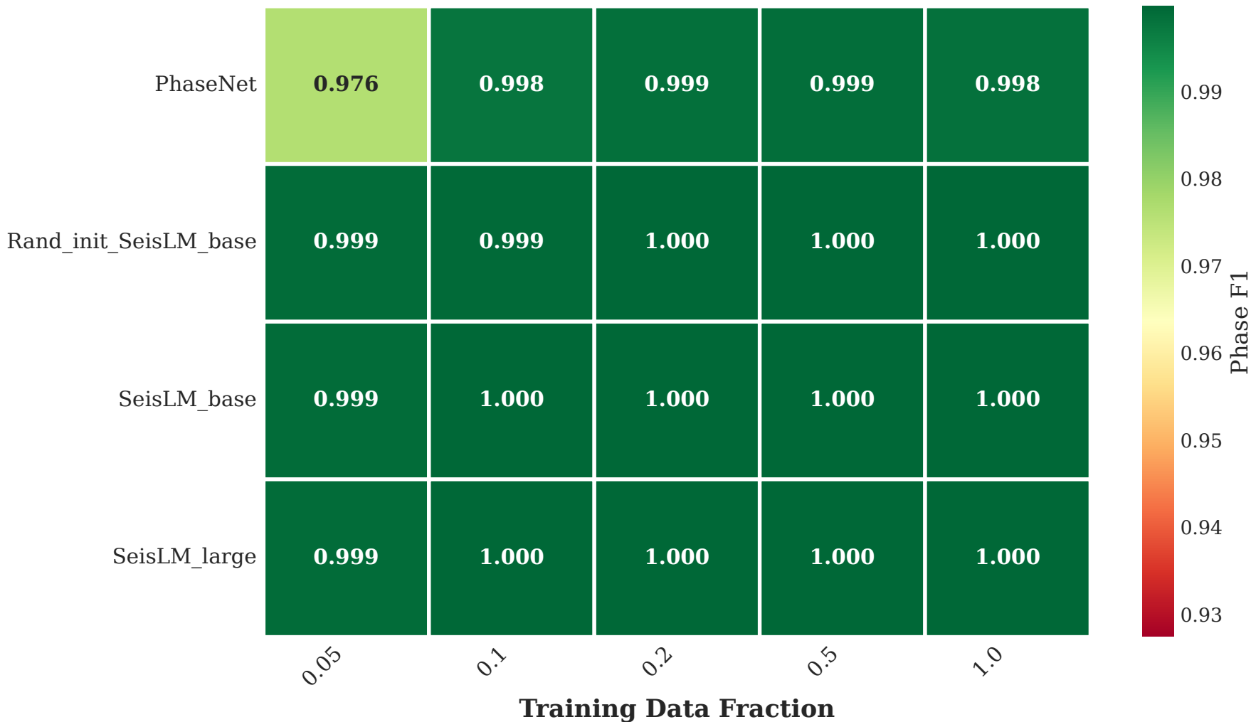
Phase Identification F1 Score - STEAD
