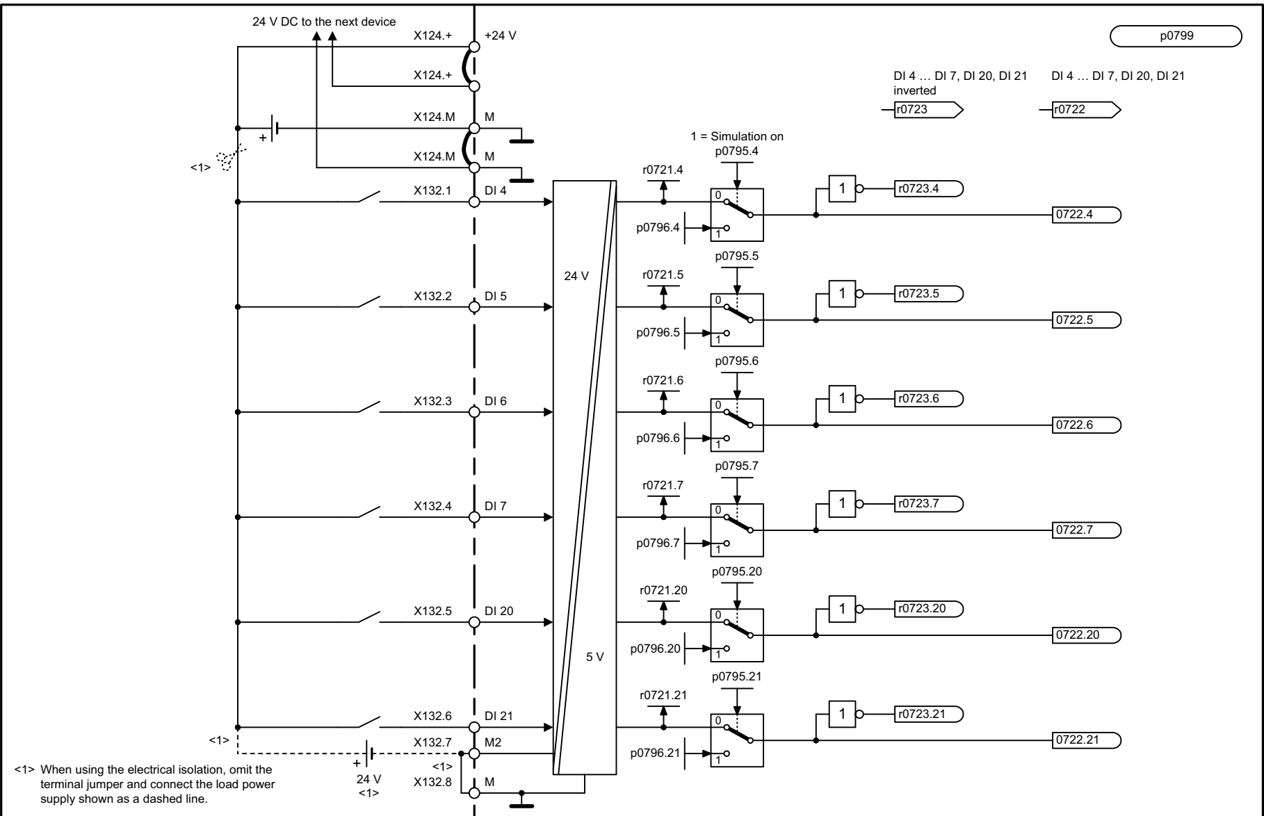
Fig. 2-17 2121 – Digital inputs, isolated (DI 4 to DI 7, DI 20, DI 21)
