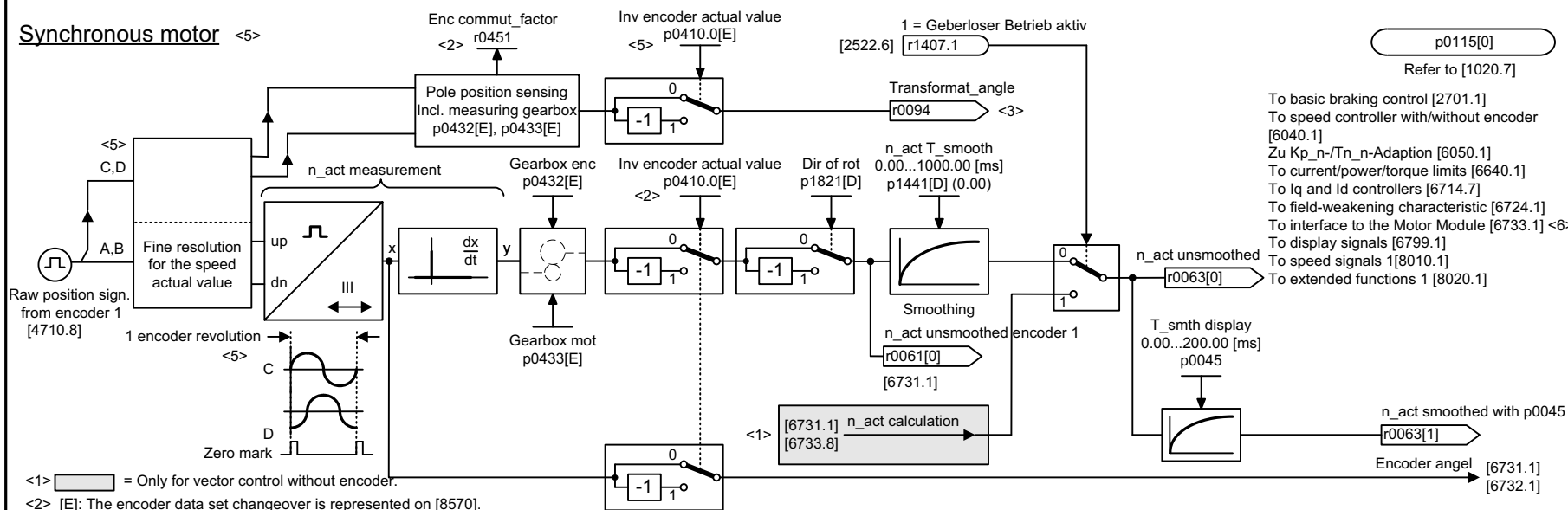
4715 – Actual speed value and pole pos. sens., motor enc. ASM/SM (encoder 1)
