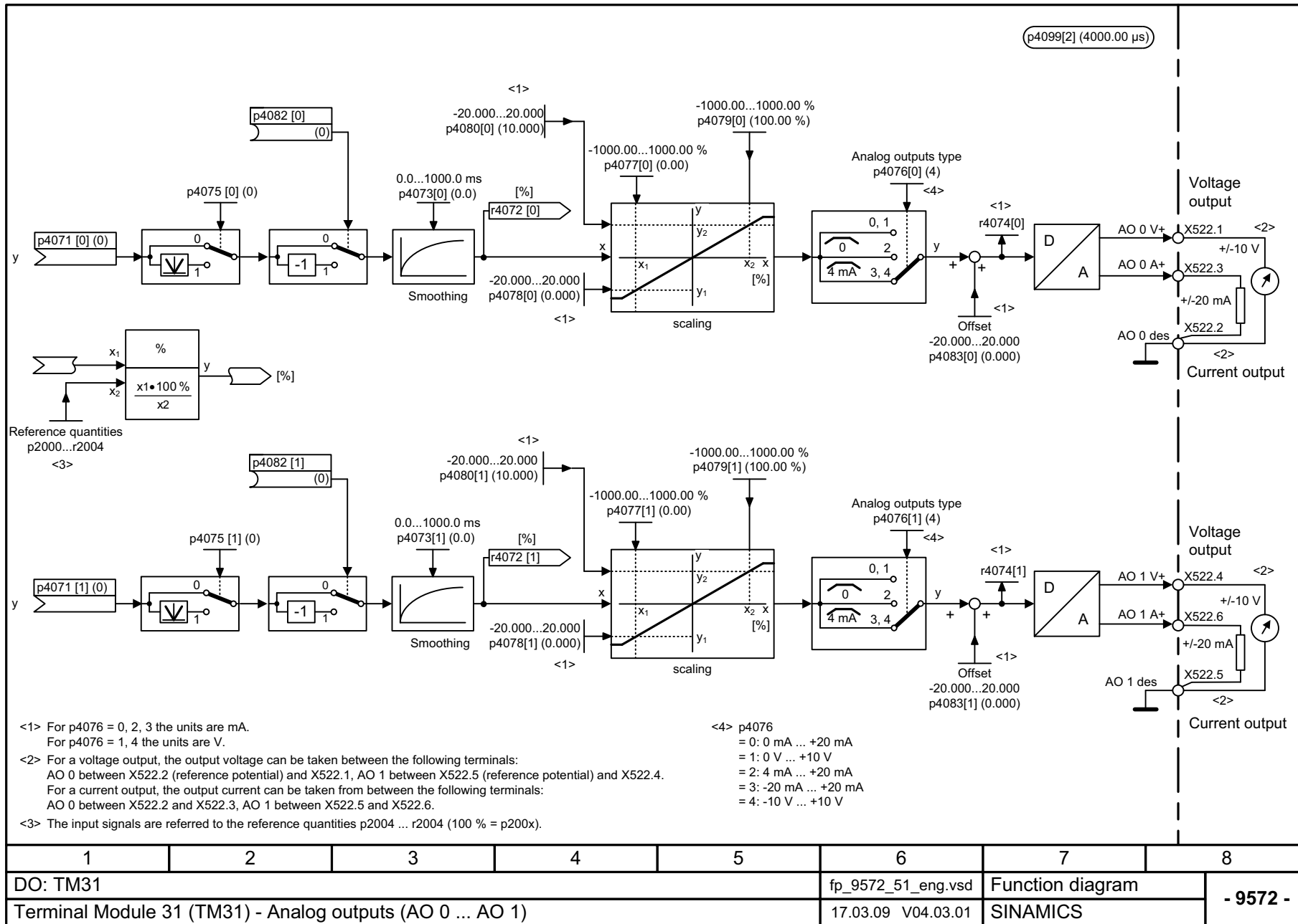
Fig. 2-151 9572 – Analog outputs (AO 0 to AO 1)
