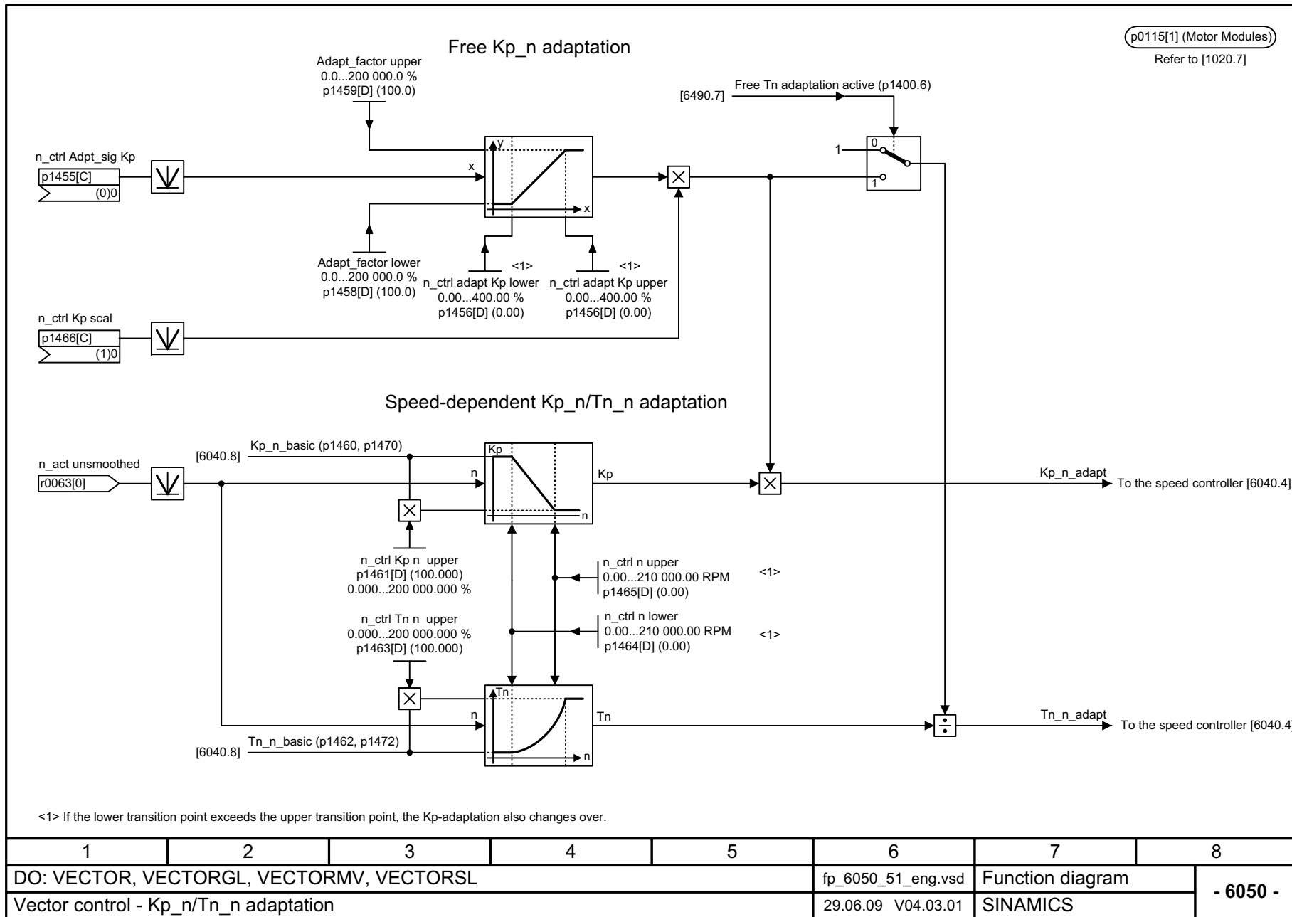
Fig. 2-88 6050 – Kp_n-/Tn_n adaptation
