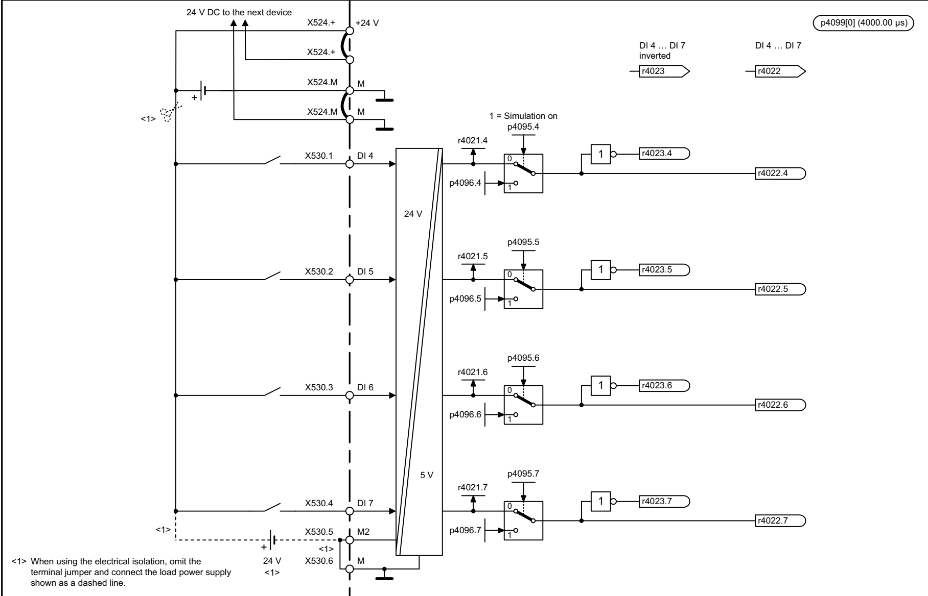
Fig. 2-145 9552 – Digital inputs, isolated (DI 4 to DI 7)
