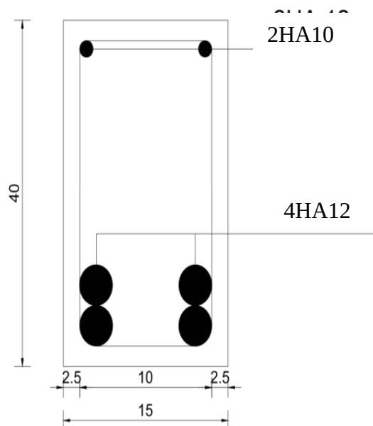
Plan de ferrailage des poutres
