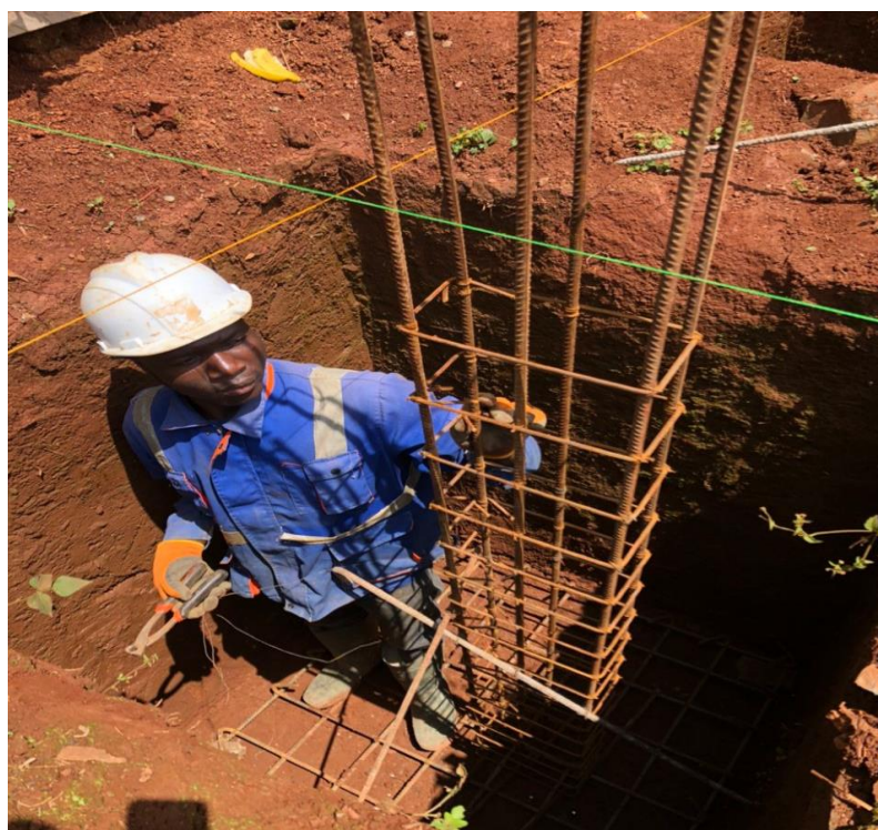
Mise en place de la semelle et amorce
