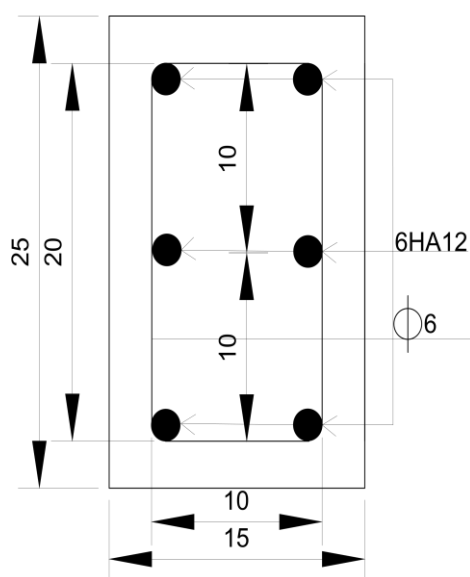
Plan de ferrailage des amorcés et poteau
