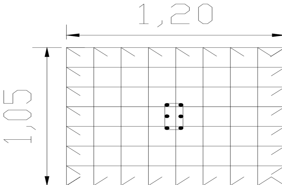
Figure 4 : Schéma de ferrailage de la semelle
