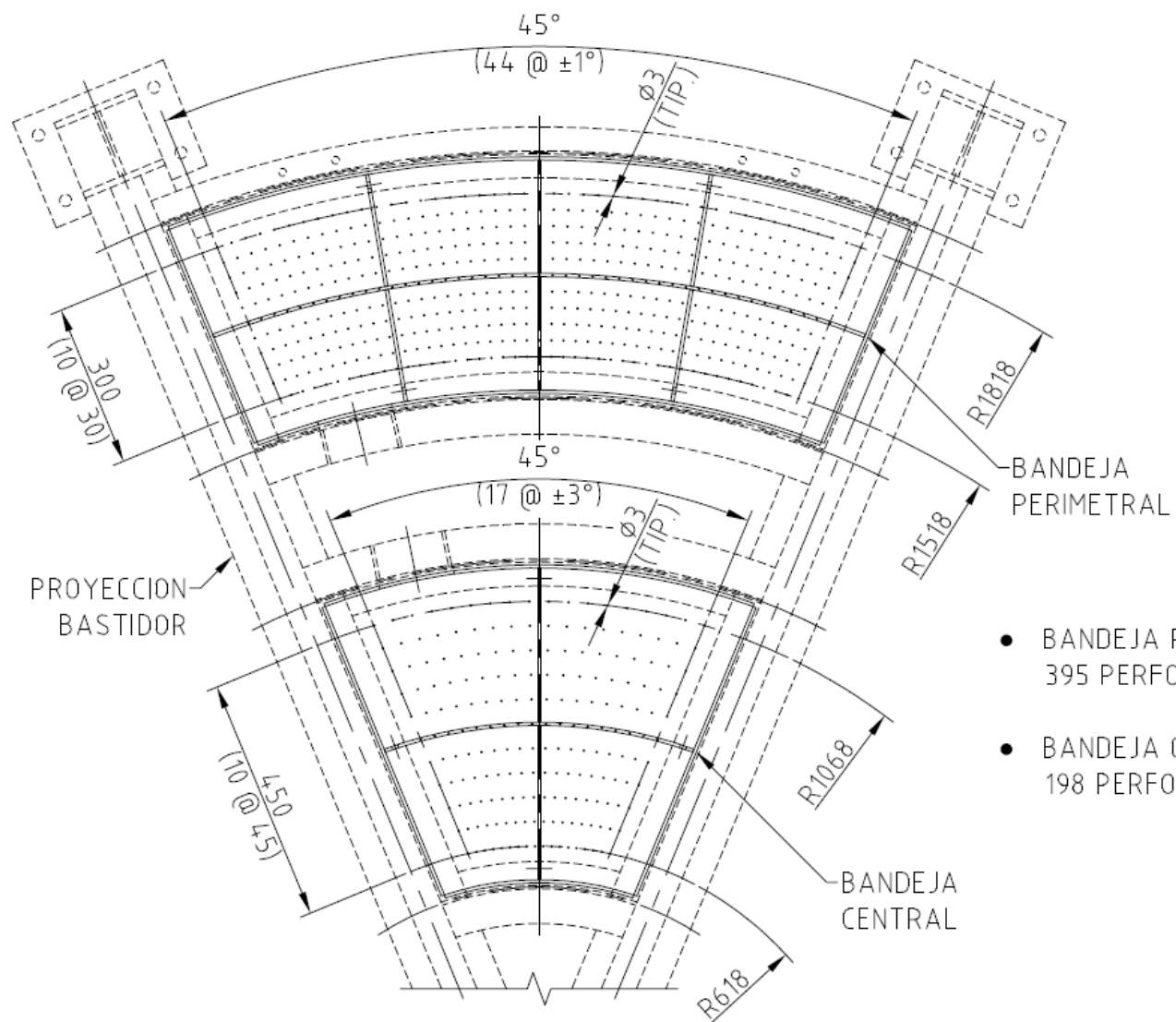
ESQUEMA PERFORACIONES BANDEJAS ESC. 1/20
